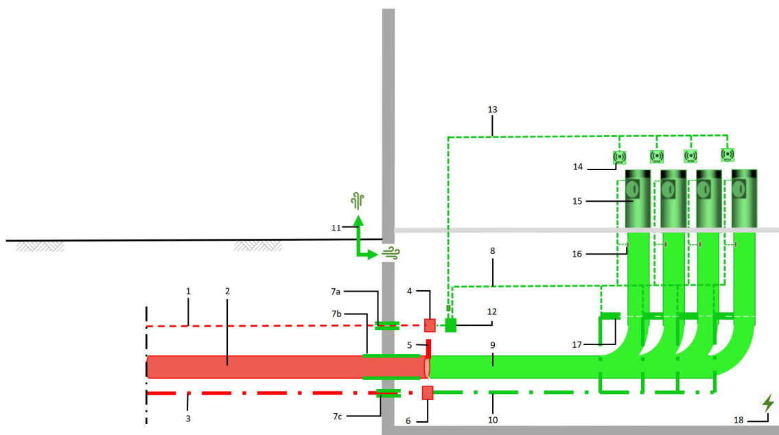
Figuur 1 Demarcatie OAT exploitant (rood) en gebouweigenaar (groen)
