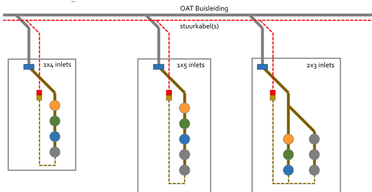
Figuur 2 Schematische indeling binneninstallatie op OAT Inzamelpunt
