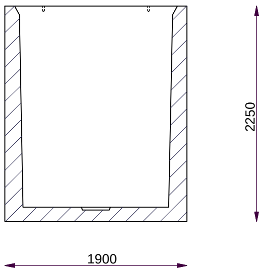
B-B ( 1 : 40 )
