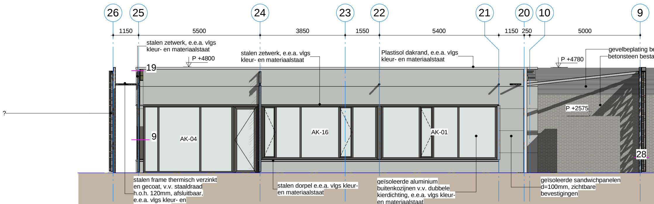
Gevel D (Westgevel nieuw)
