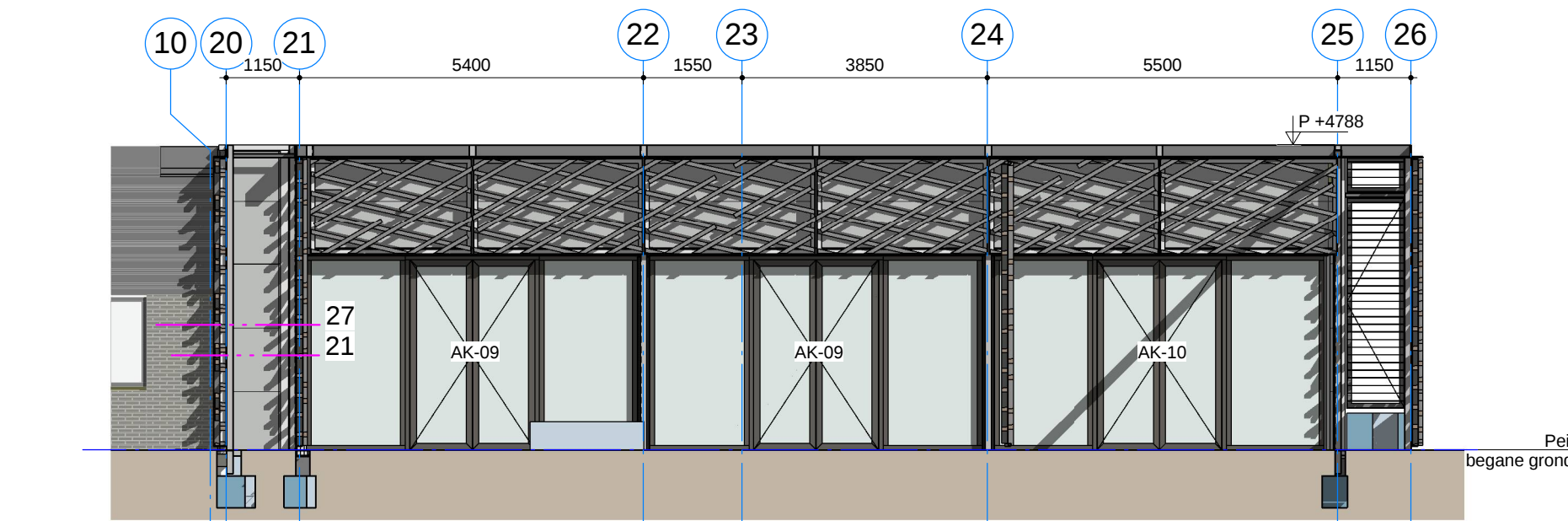
Gevel B' (Oostgevel kantoor nieuw - achter scherm)
