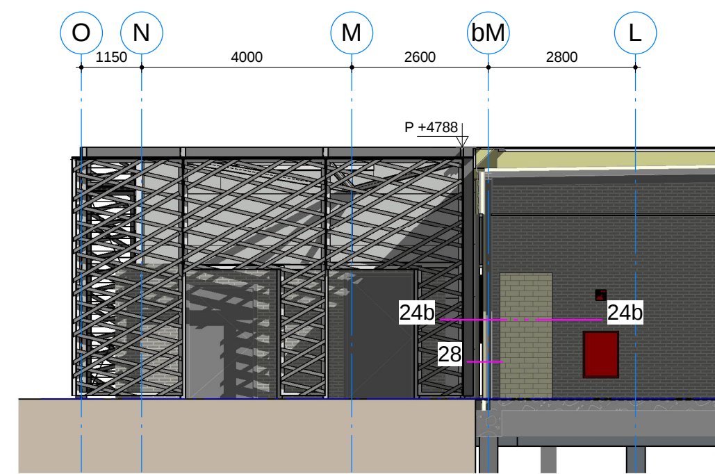
Gevel F (Zuidgevel nieuw traforuimte)
