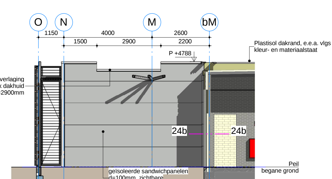
Gevel H (Zuidgevel kantoor nieuw - achter scherm)
