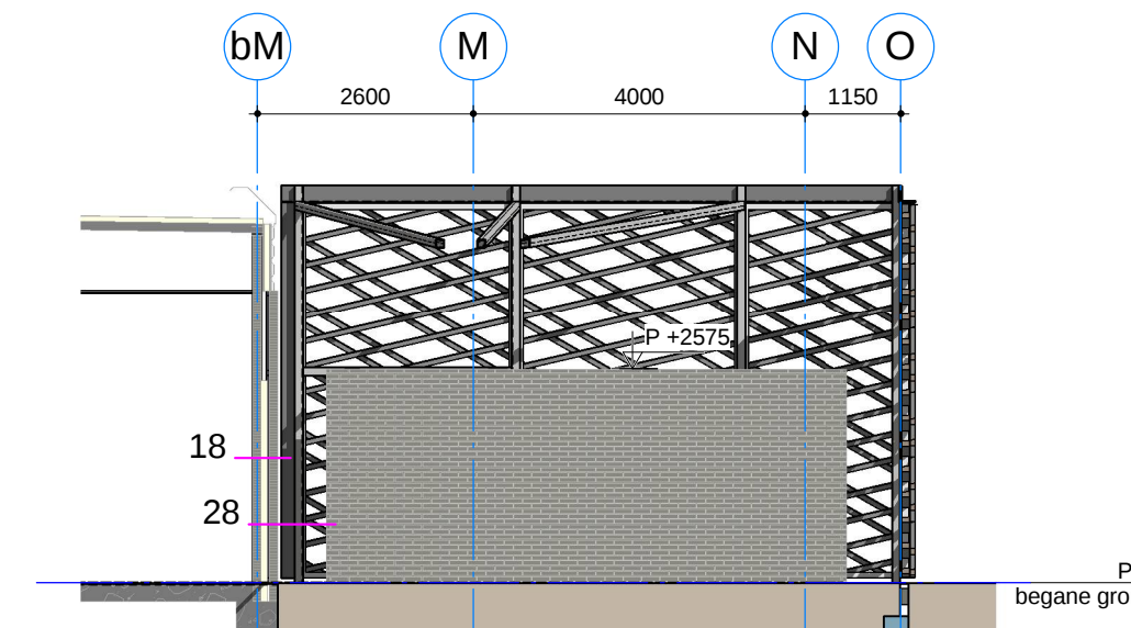
Gevel G (Noordgevel nieuw traforuimte)
