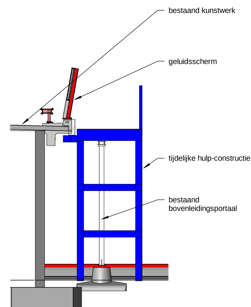
doorsnede hulp-constructie nieuwe situatie
