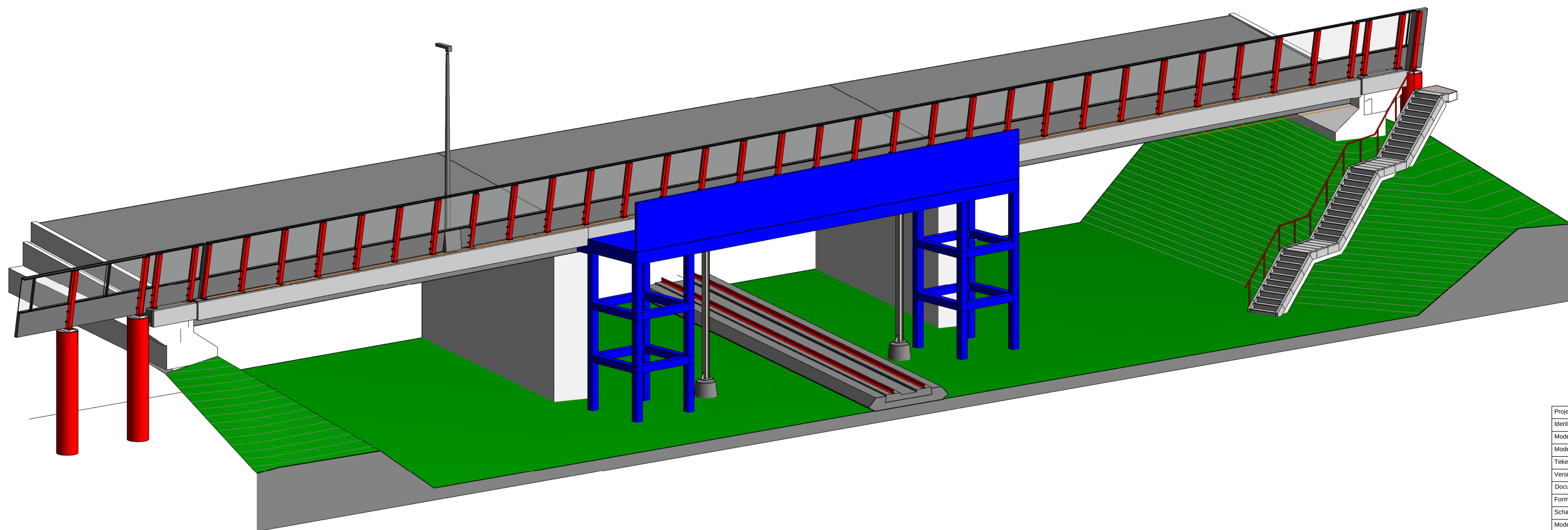
3D bestaand kunstwerk met geluidsscherm en hulp-constructie
