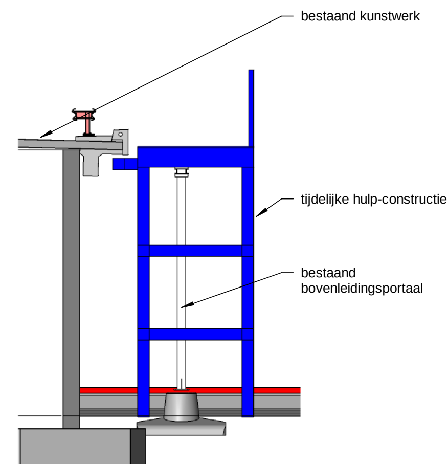
doorsnede hulp-constructie bestaande situatie
