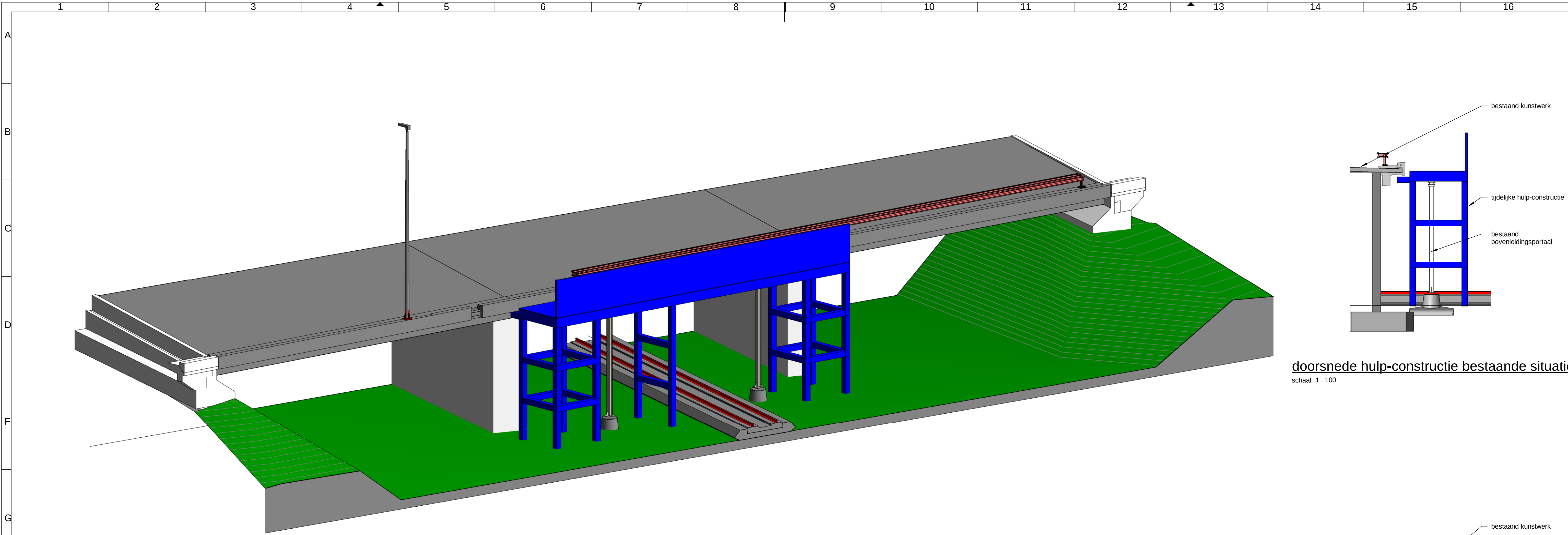
3D bestaand kunstwerk met hulp-constructie
