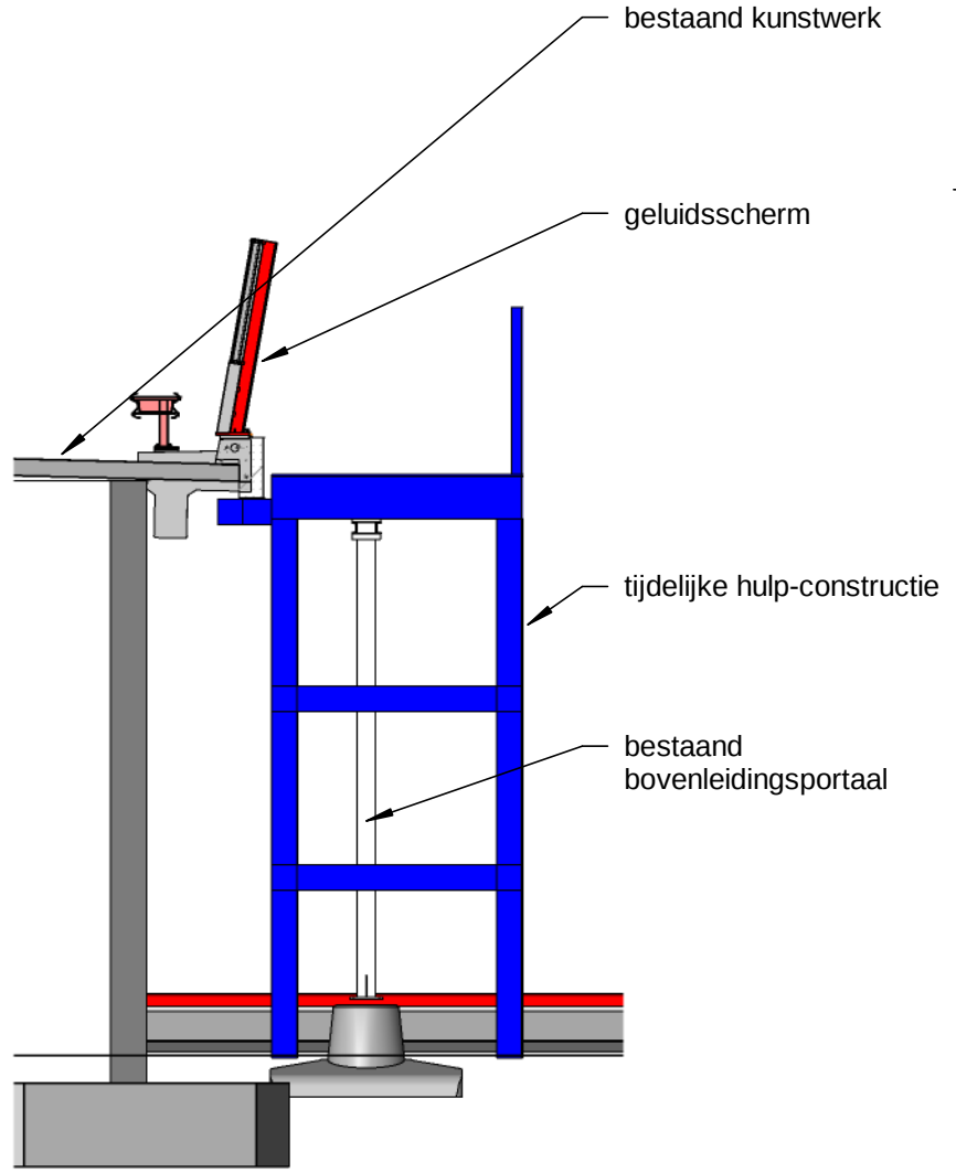
doorsnede hulp-constructie nieuwe situatie schaal: 1 : 100
