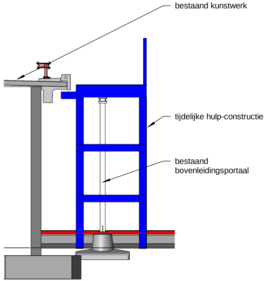
doorsnede hulp-constructie bestaande situatie schaal: 1 : 100
