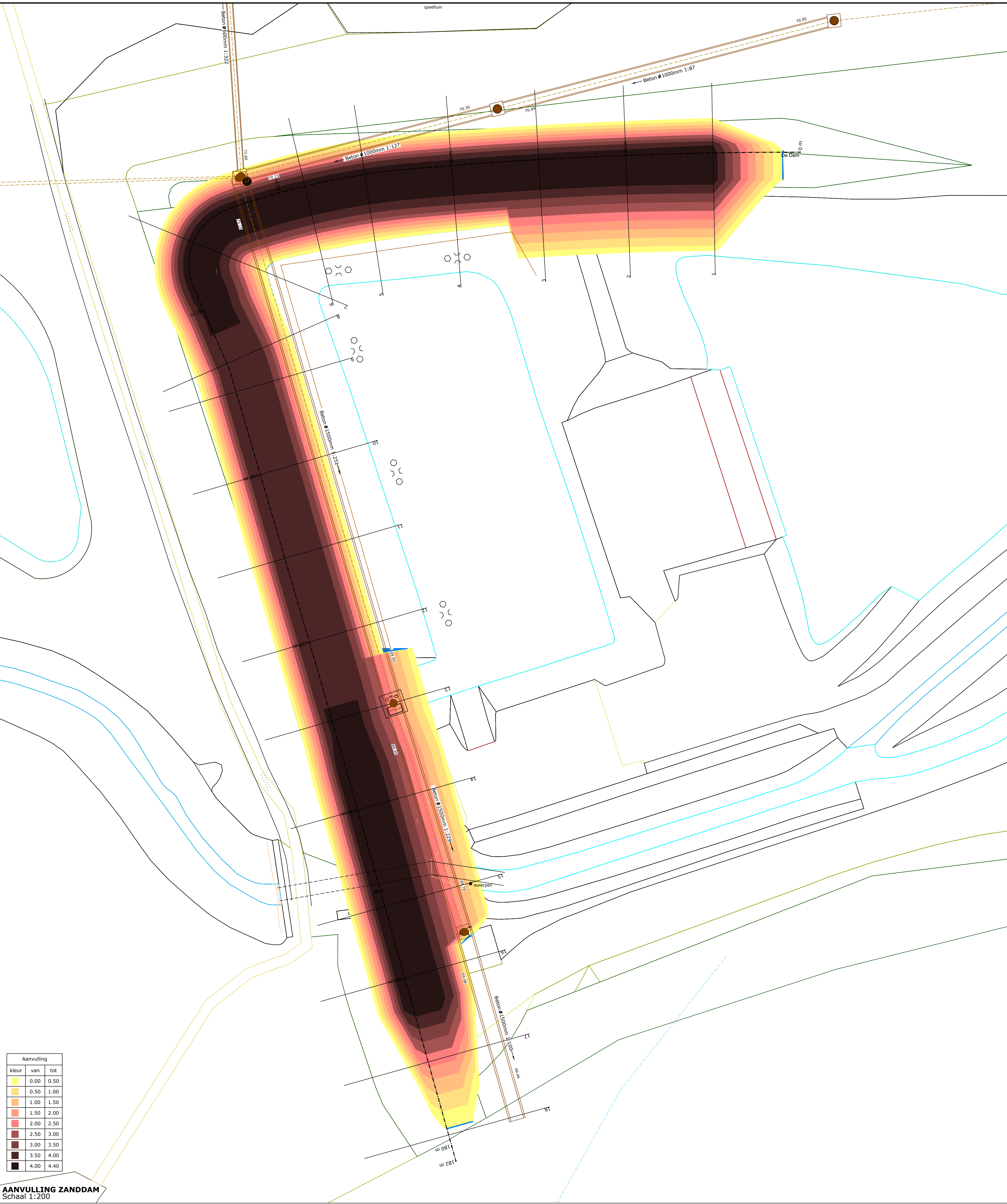
EINDSITUATIE Schaal 1:200
