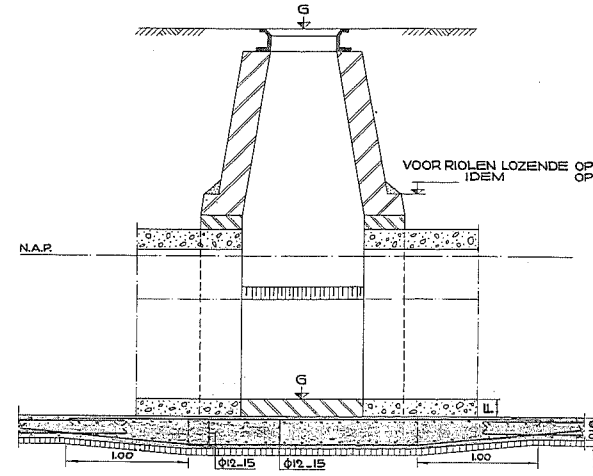
DOORSNEDE E.F.
