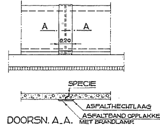
VOEGDICHTING.
