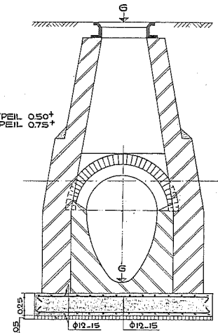
DOORSNEDE G.H.
