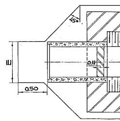
INSTEEKBUIS.
