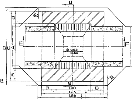
HORIZONTALE DOORSNEDE.
