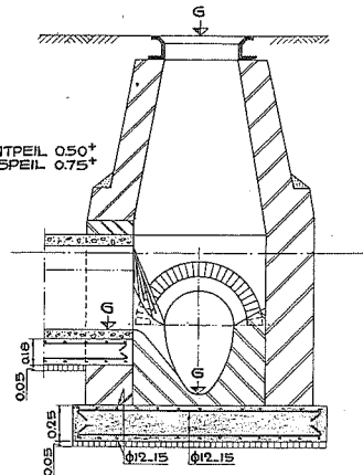
DOORSNEDE C.D.
