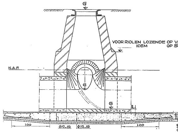
DOORSNEDE A.B.
