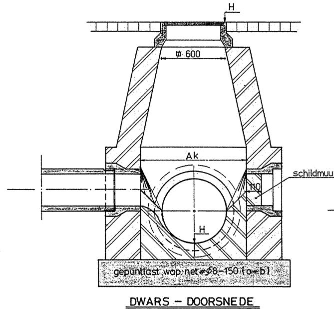
INSPECTIEPUT BIJ KRUISEND RIOOL
