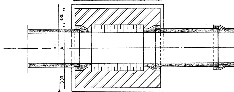
HORIZONTALE DOORSNEDE
