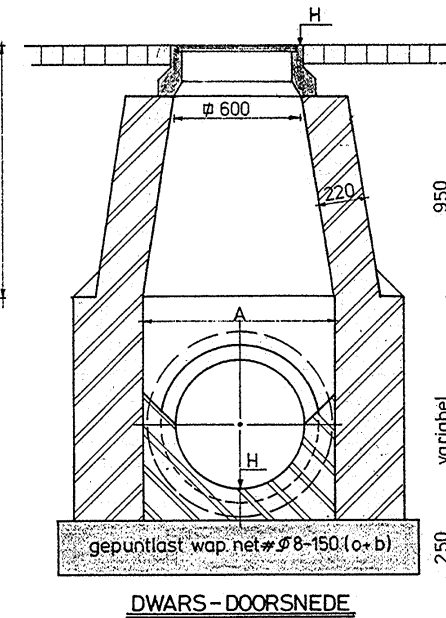
INSPECTIEPUT BIJ DOORGAAND RIOOL
