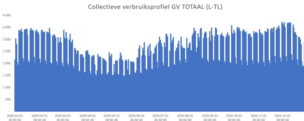
Grafiek 1: Collectieve verbruiksprofiel grootverbruik o.b.v. meetdata 2020
