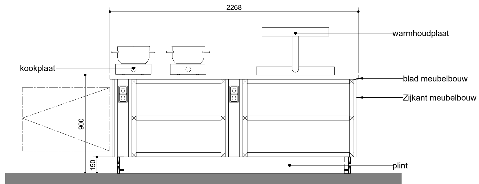
Aanzicht uitgifte buffet 509
