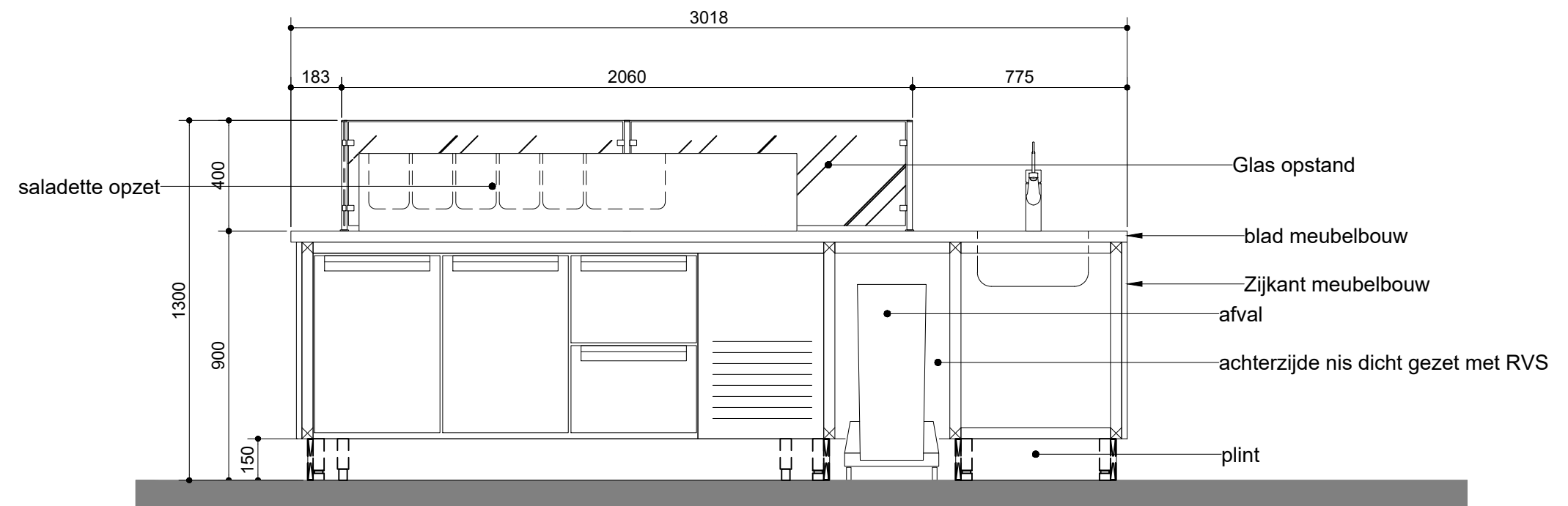
Aanzicht uitgifte buffet 501
