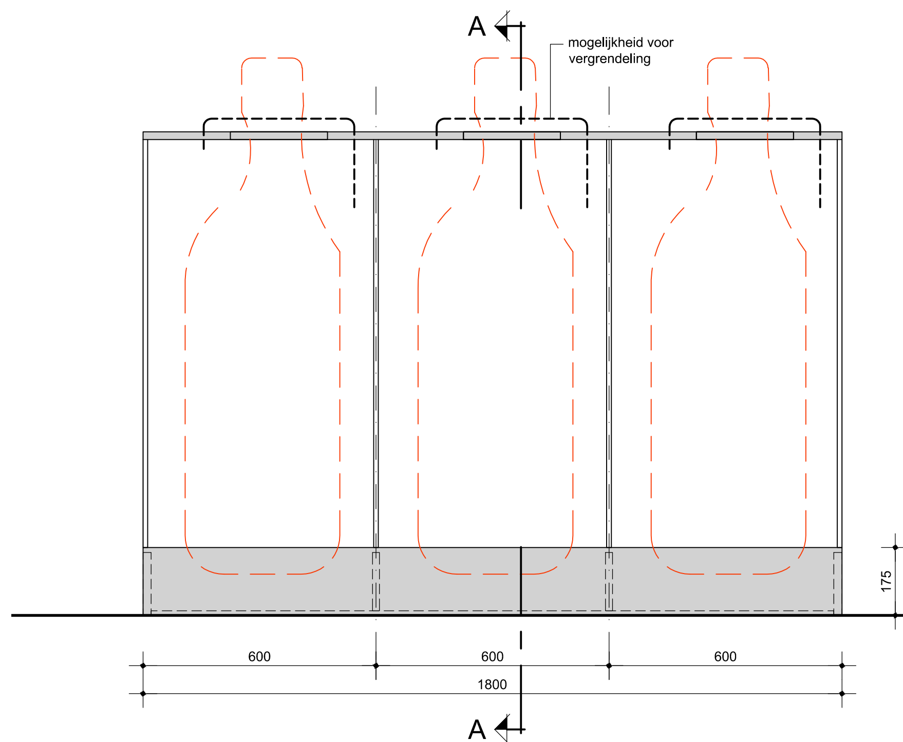
vooraanzicht
