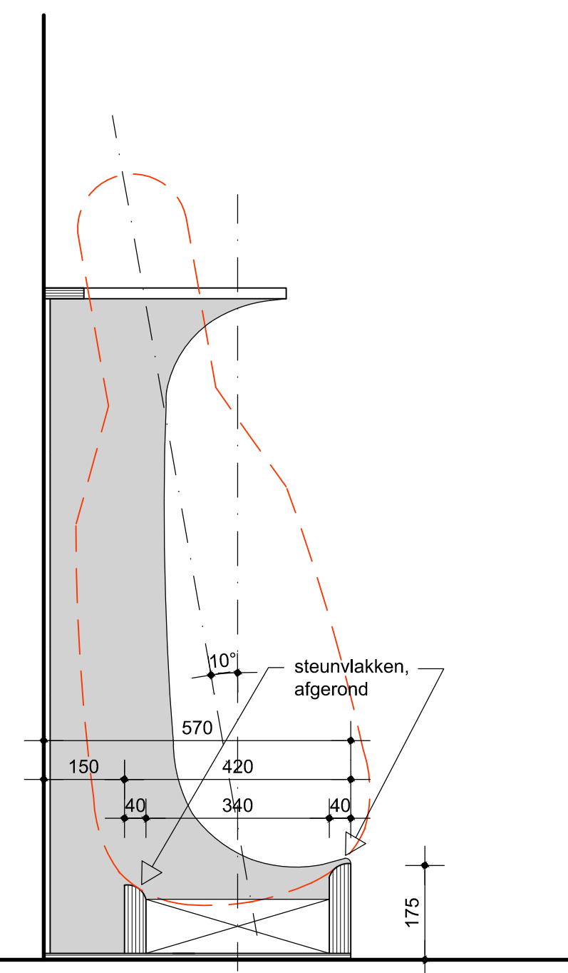
doorsnede
