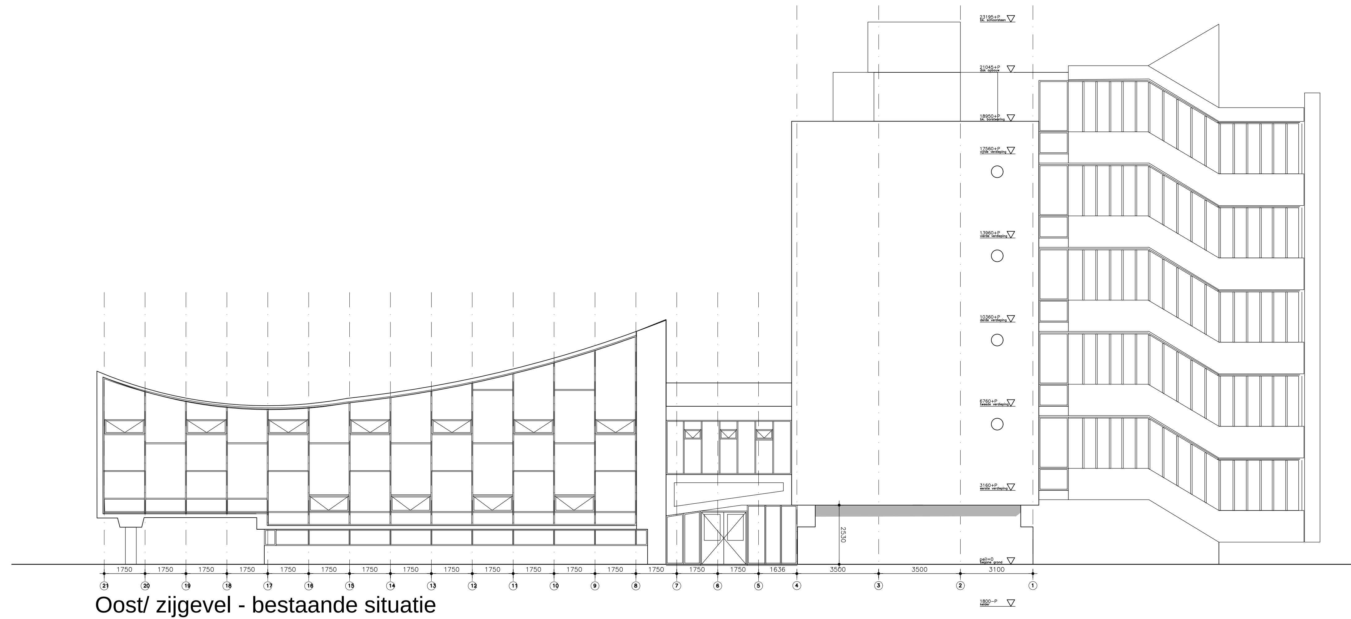
Oost/ zijgevel - bestaande situatie
