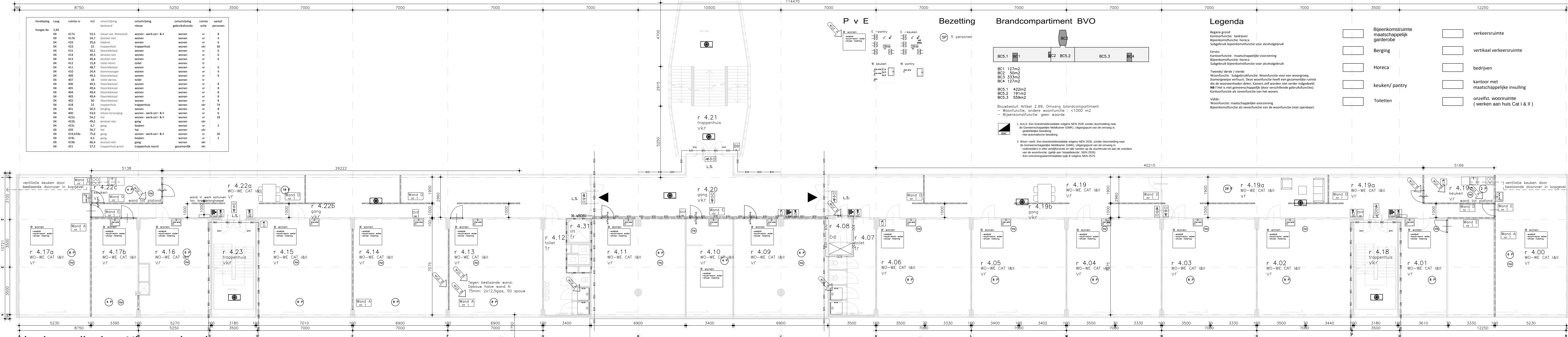
vierde verdieping Nieuwe situatie
