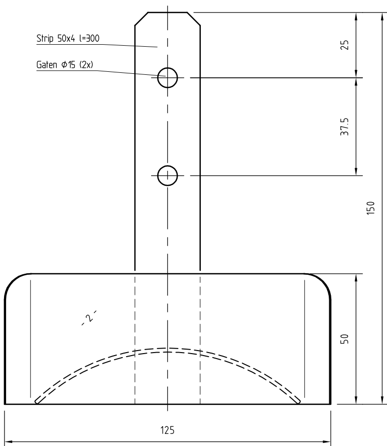
Vooraanzicht
