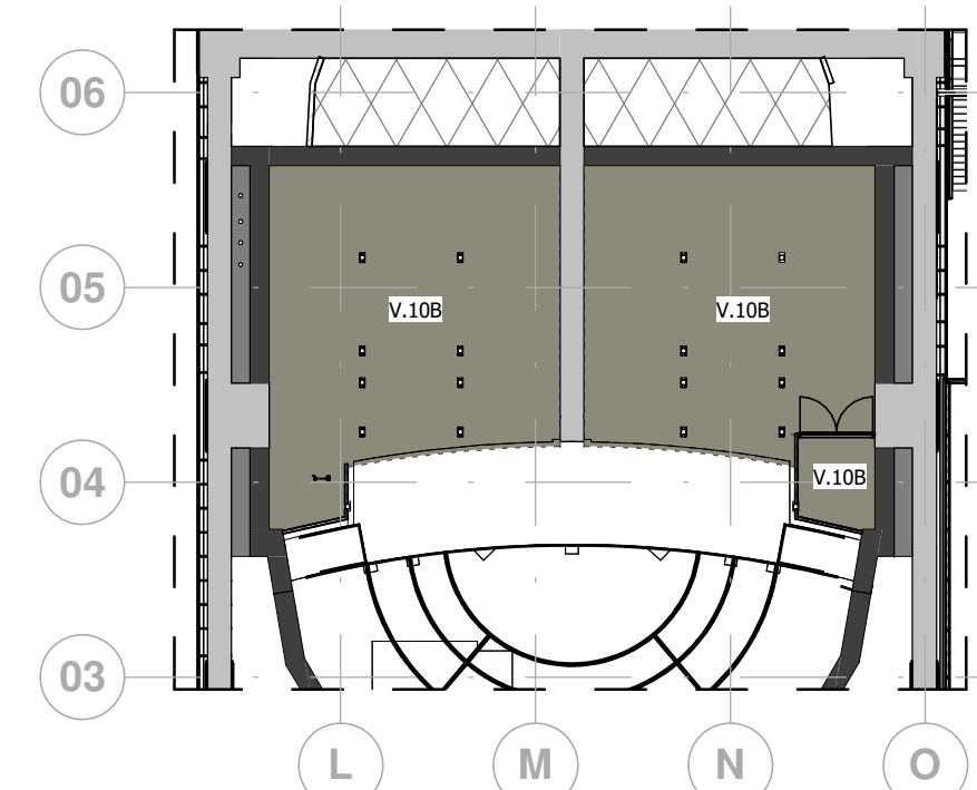
Niveau onder concertzaal
