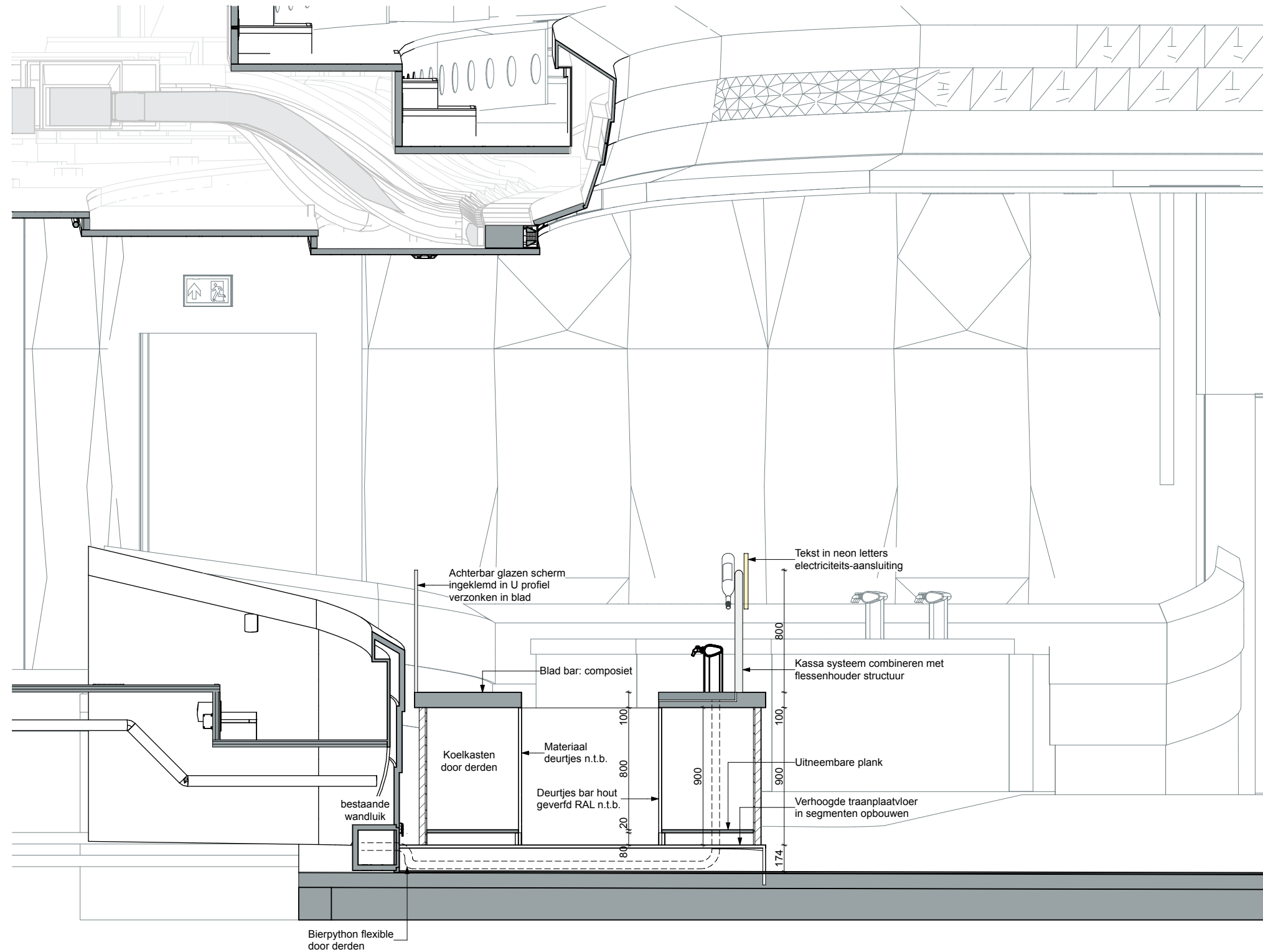
Bar types B1, B2 Doorsnede
