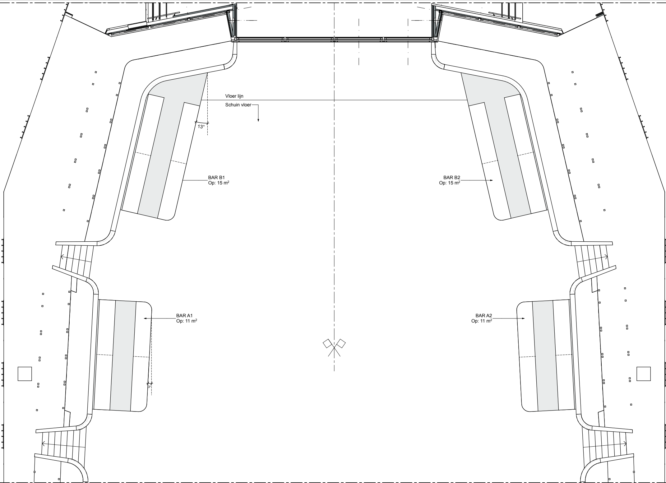
Concertzaal Popbarren Plattegrond overzicht
