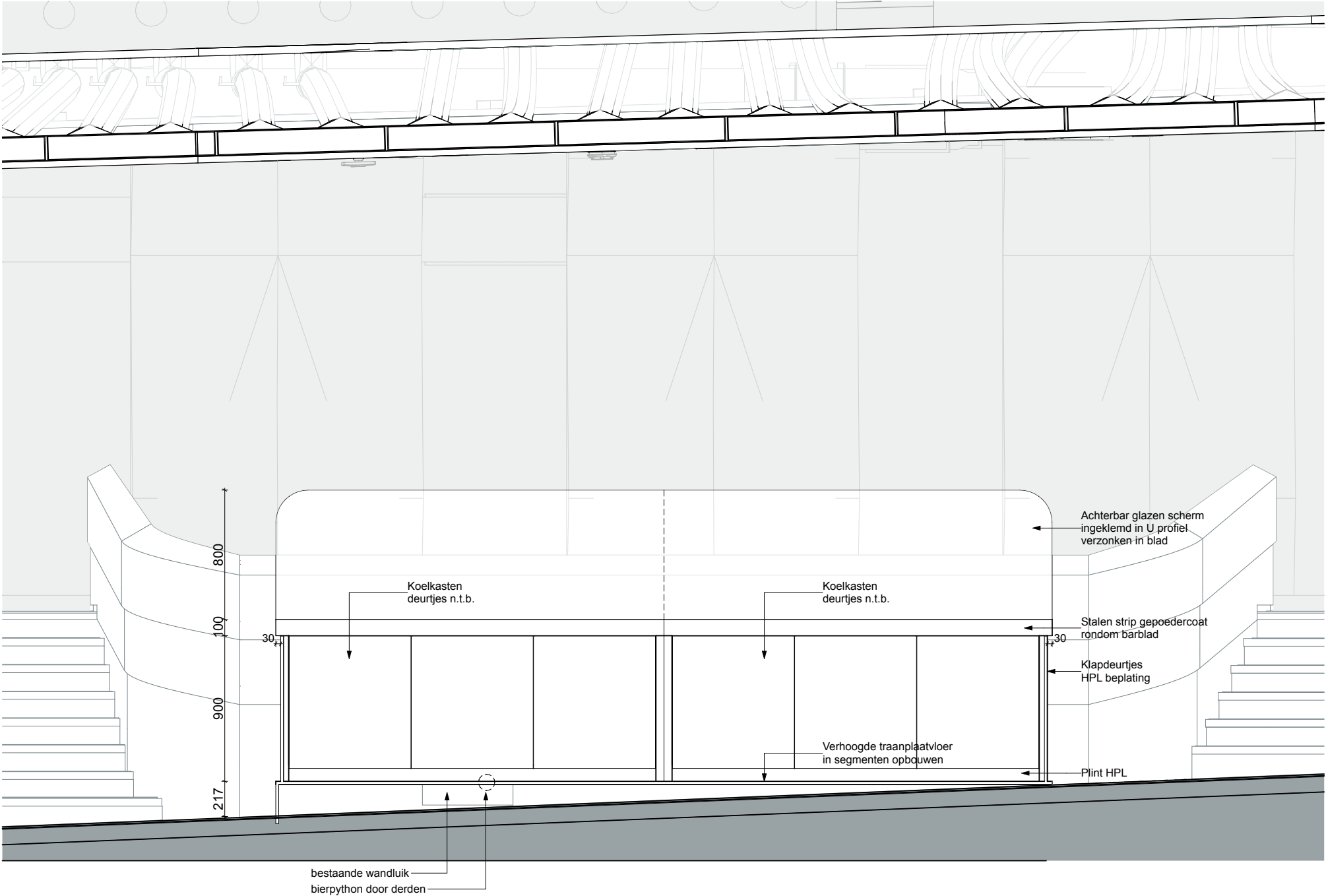
Bar types B1, B2 Aanzicht achterbar
