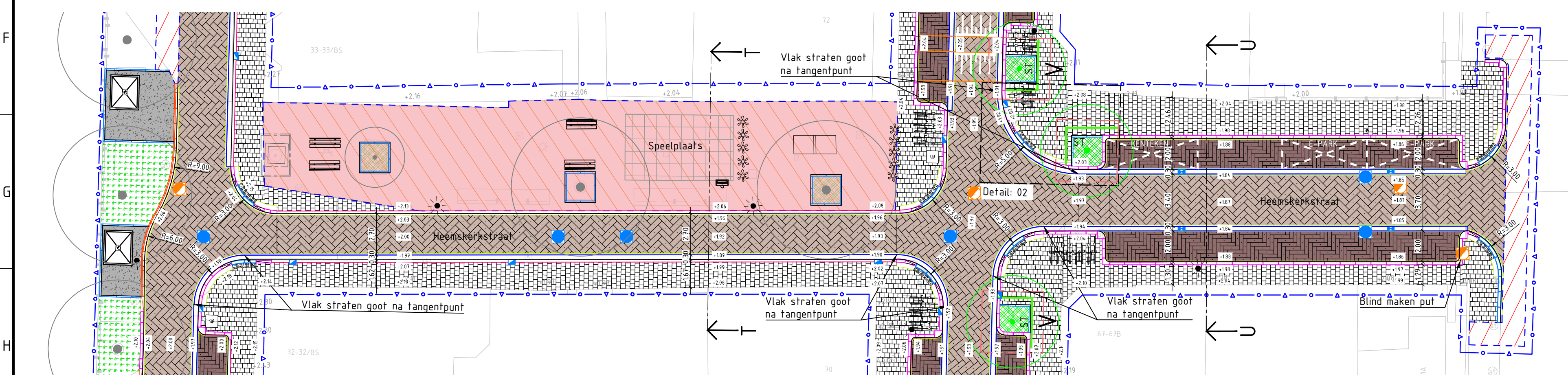
VIEW 2 SCHAAL 1 : 200
