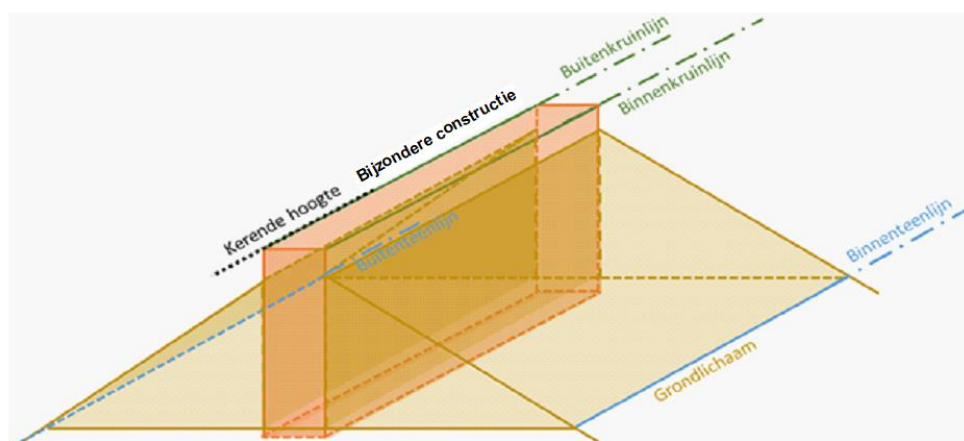
Figuur 8-11: Zijaanzicht van bijzondere constructie
