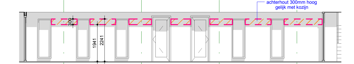
fragment aanzicht b 1:100
