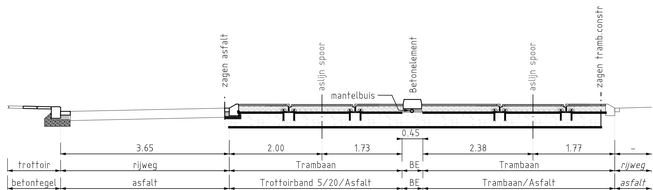
Doorsnede H-H Schaal 1:50
