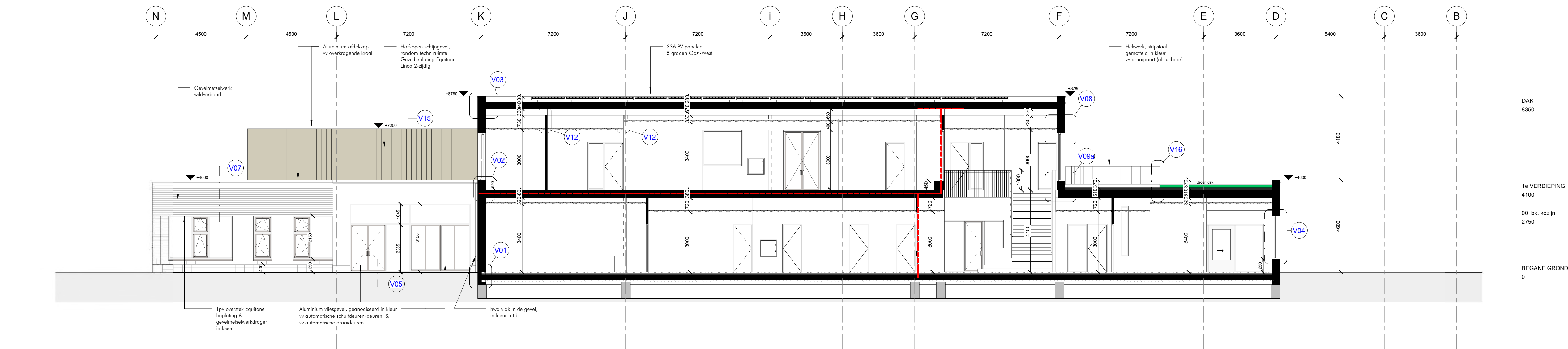
Doorsnede C schaal 1 : 100
