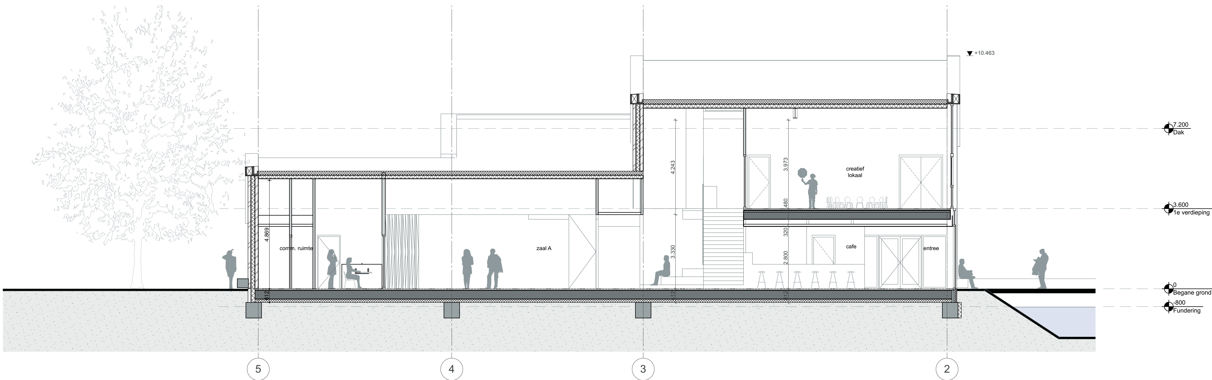
doorsnede C-C
