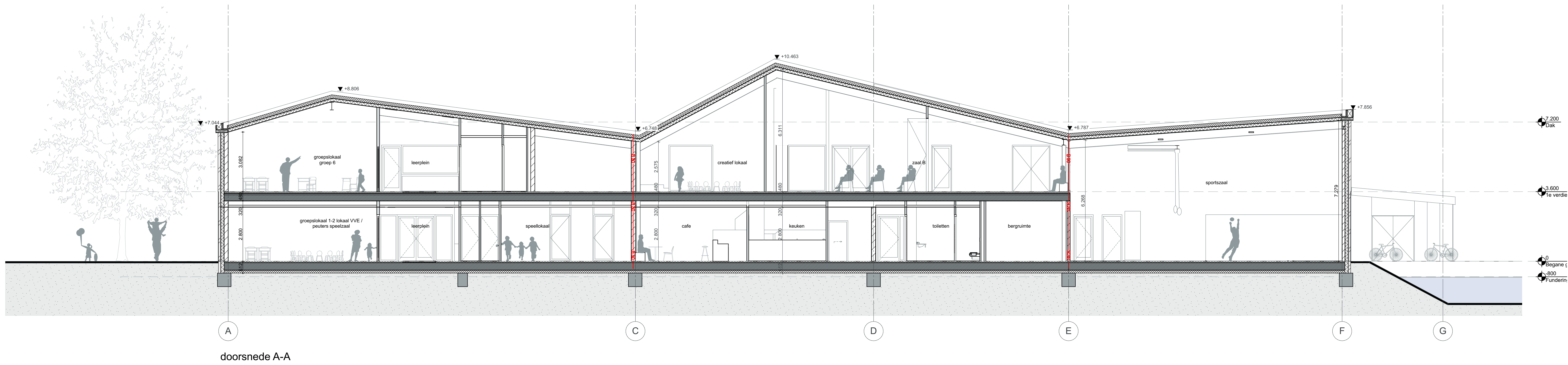
doorsnede A-A
