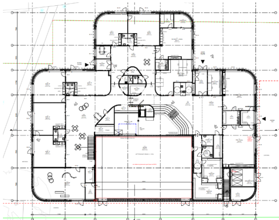
Plattegrond
