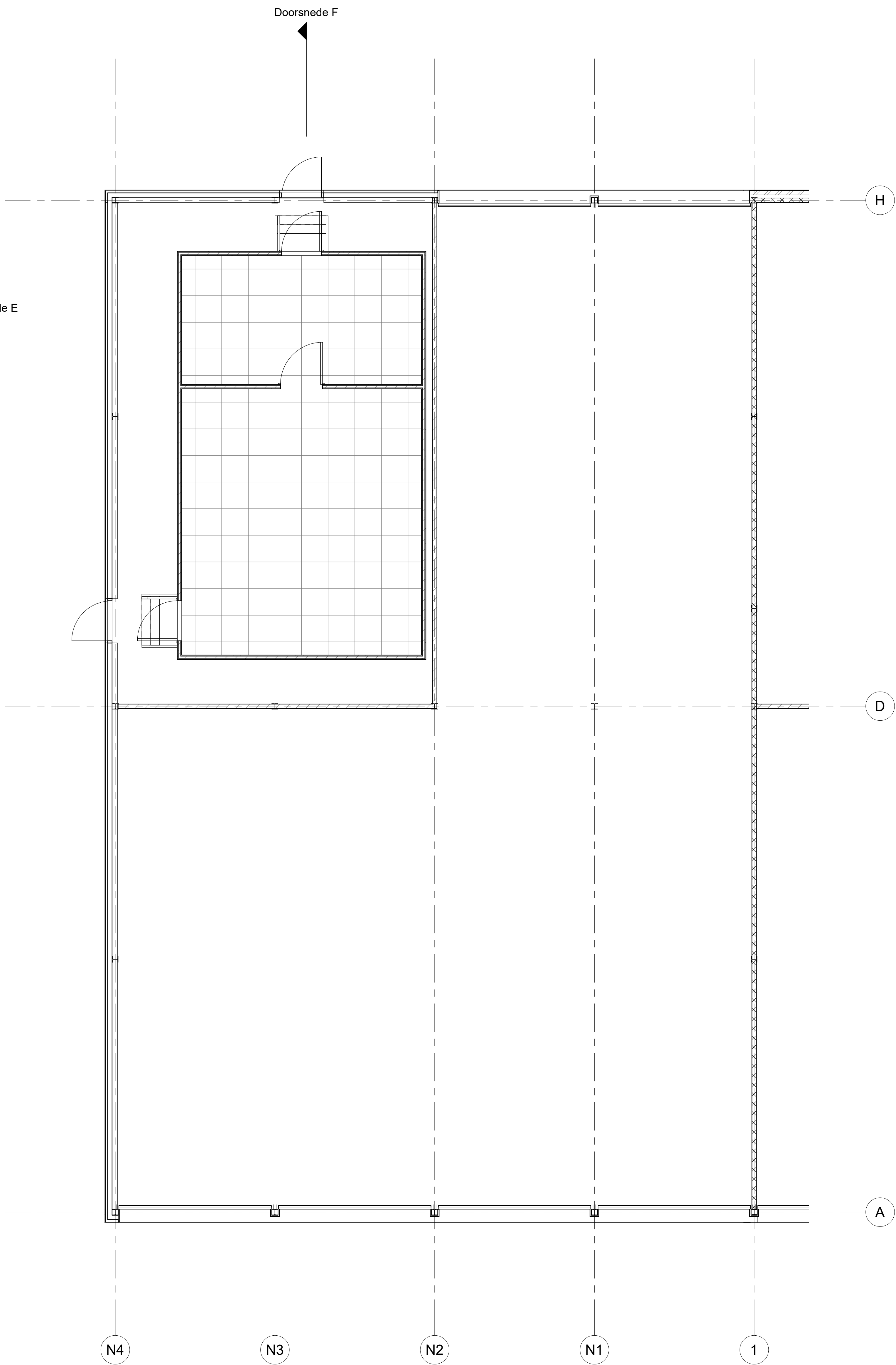
BEGANE GROND - 1:50 nieuwe situatie
