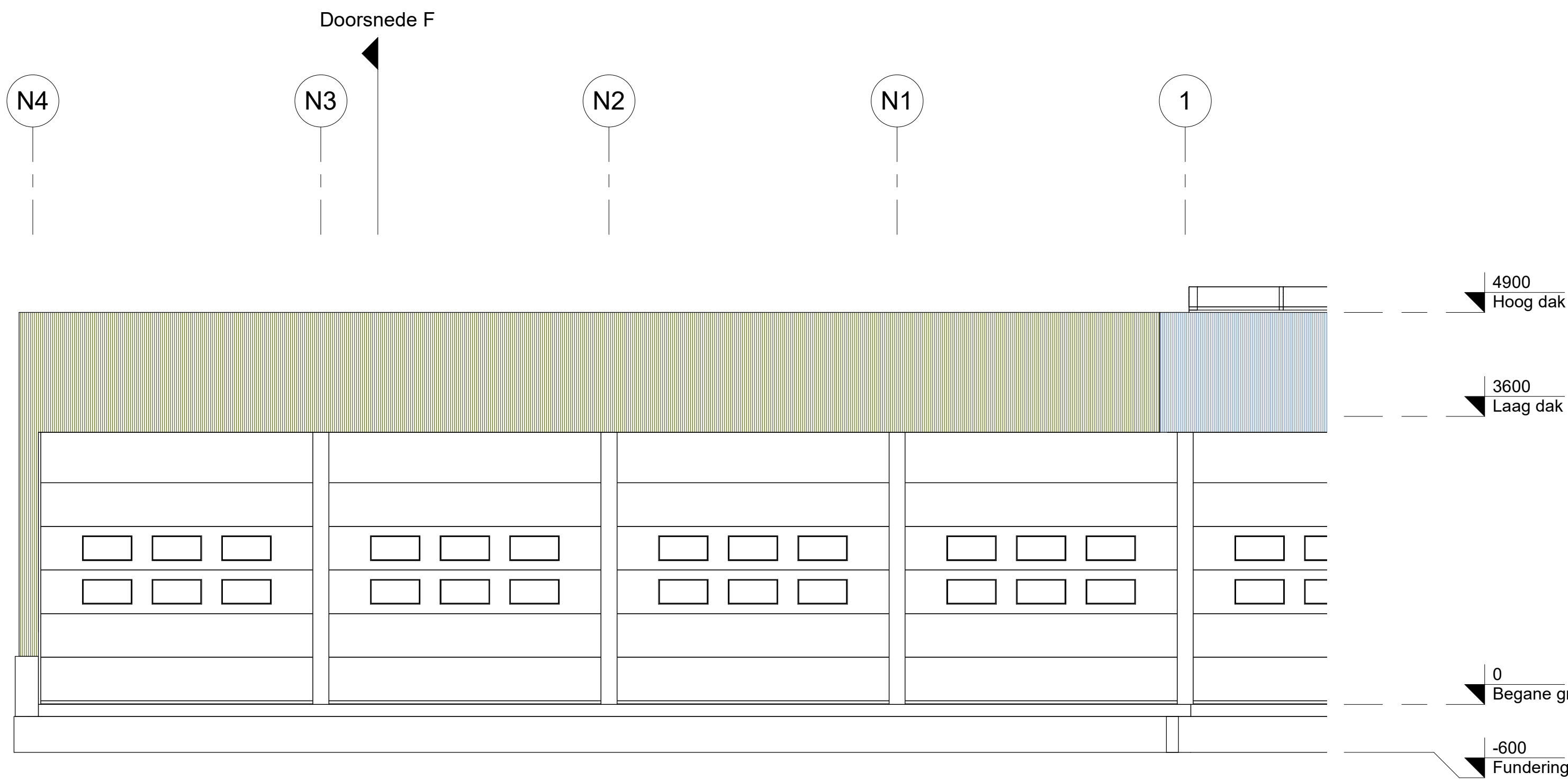
VOORGEVEL - 1:50 nieuwe situatie
