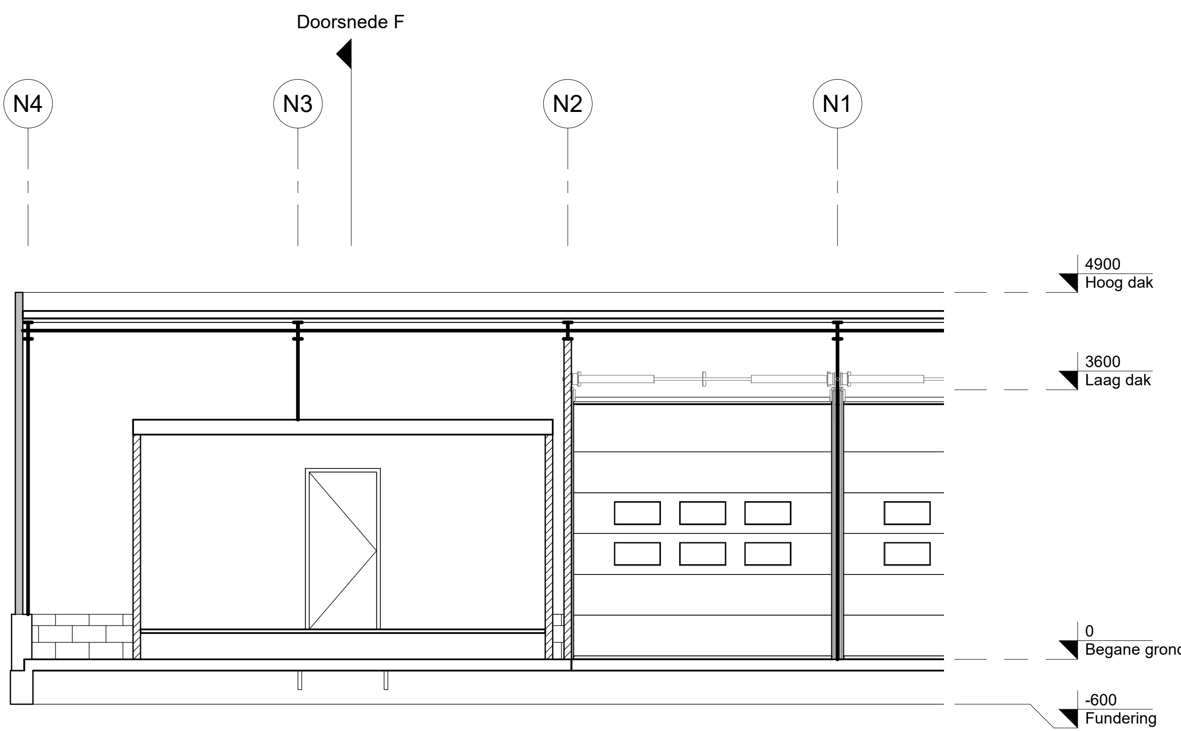
DOORSNEDE E - 1:50 nieuwe situatie
