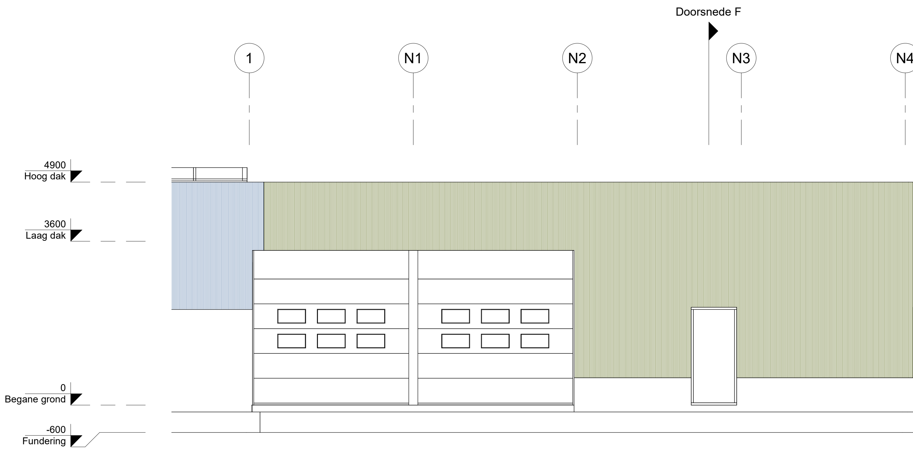
ACHTERGEVEL - 1:50 nieuwe situatie
