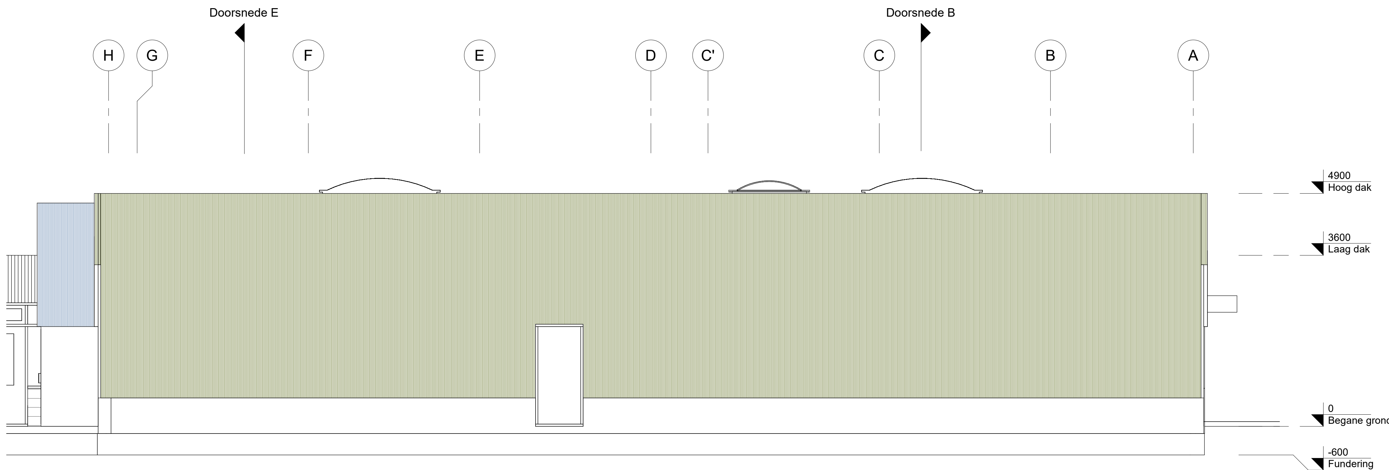
LINKER ZIJGEVEL - 1:50 nieuwe situatie
