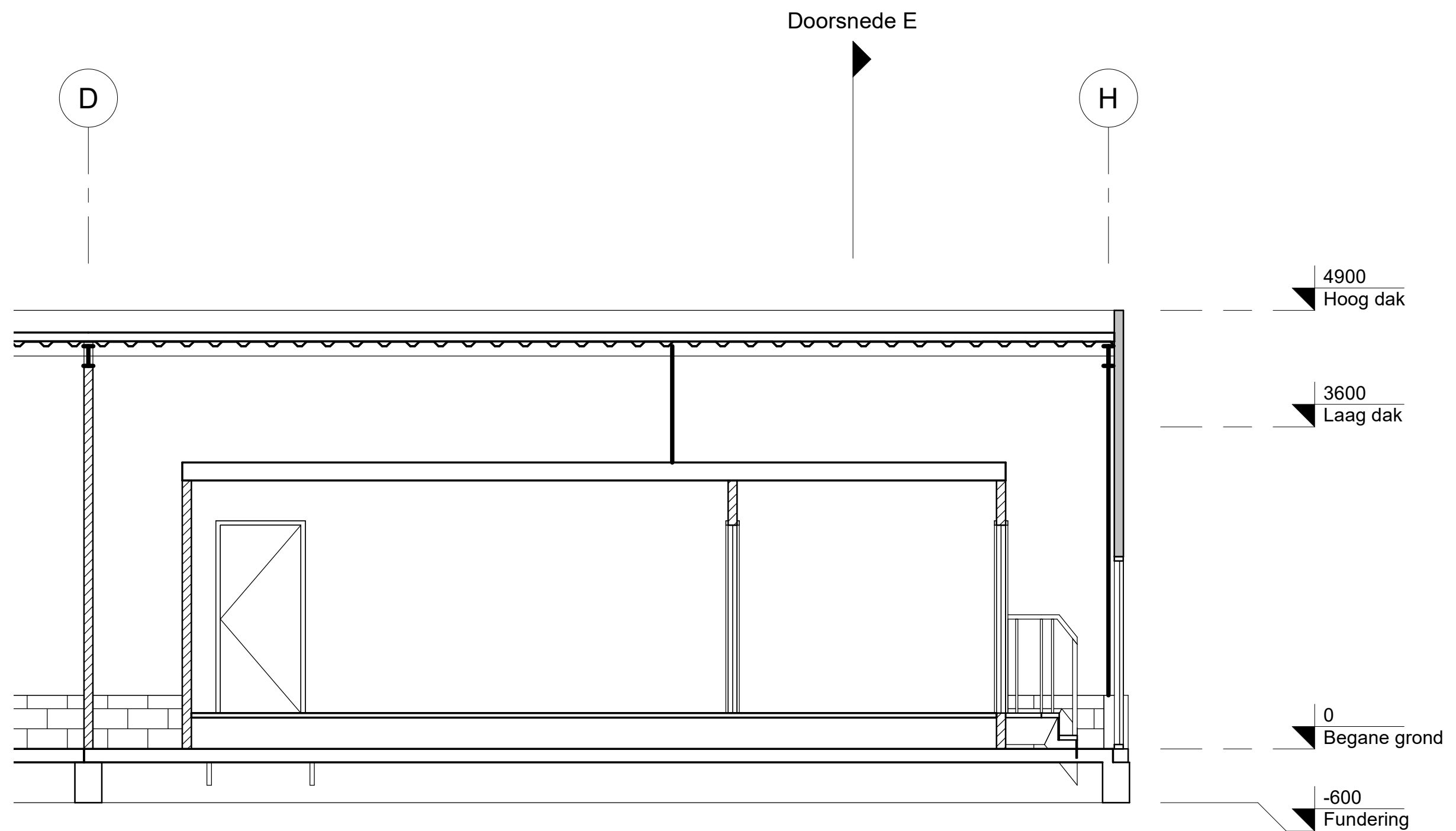
DOORSNEDE F - 1:50 nieuwe situatie
