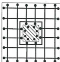
Bovenaanzicht inpakwapening hsp rond heipalen. sch.:1:20 Doorsnede B_B
