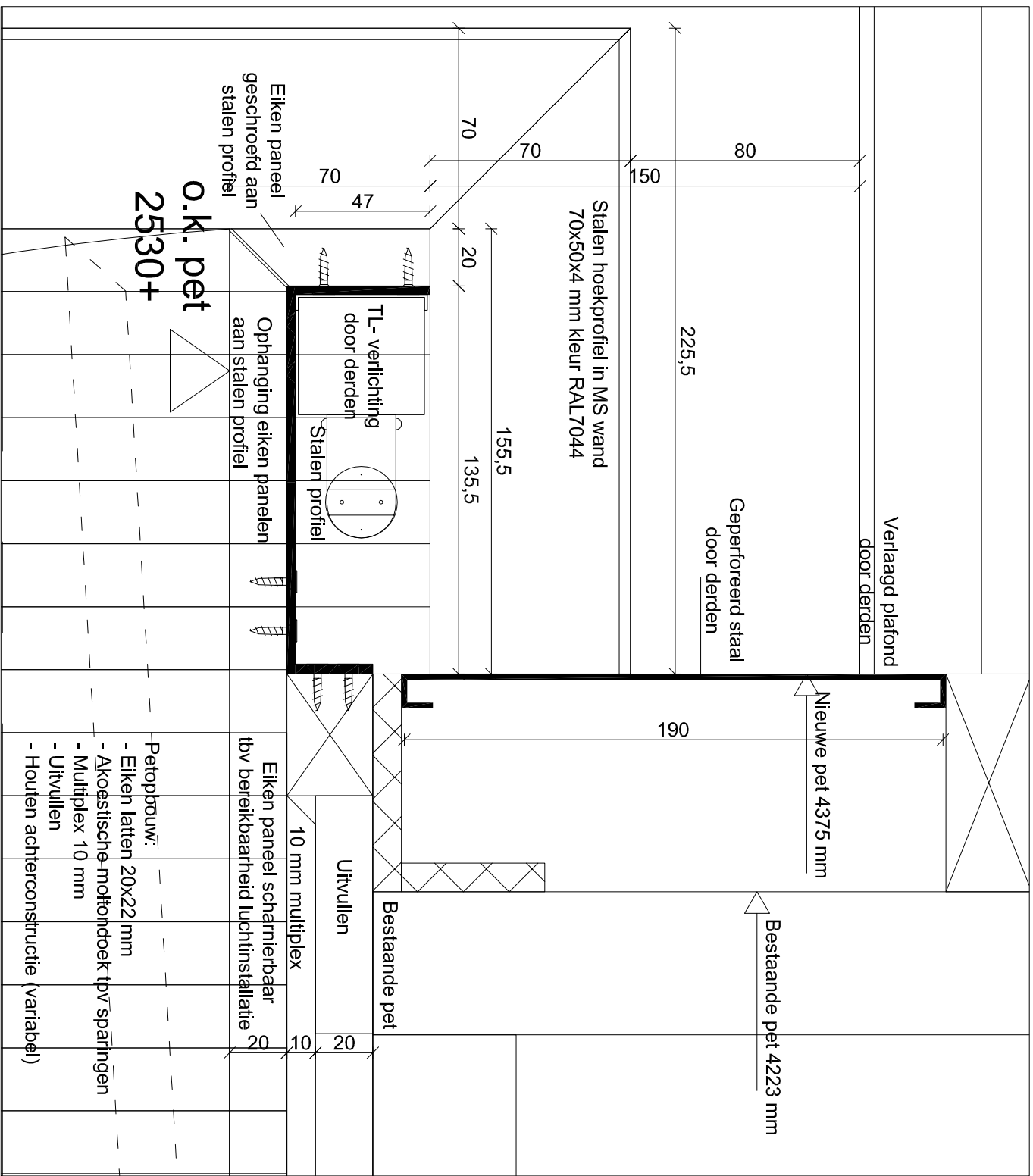
Detail A (schaal 1:2)
