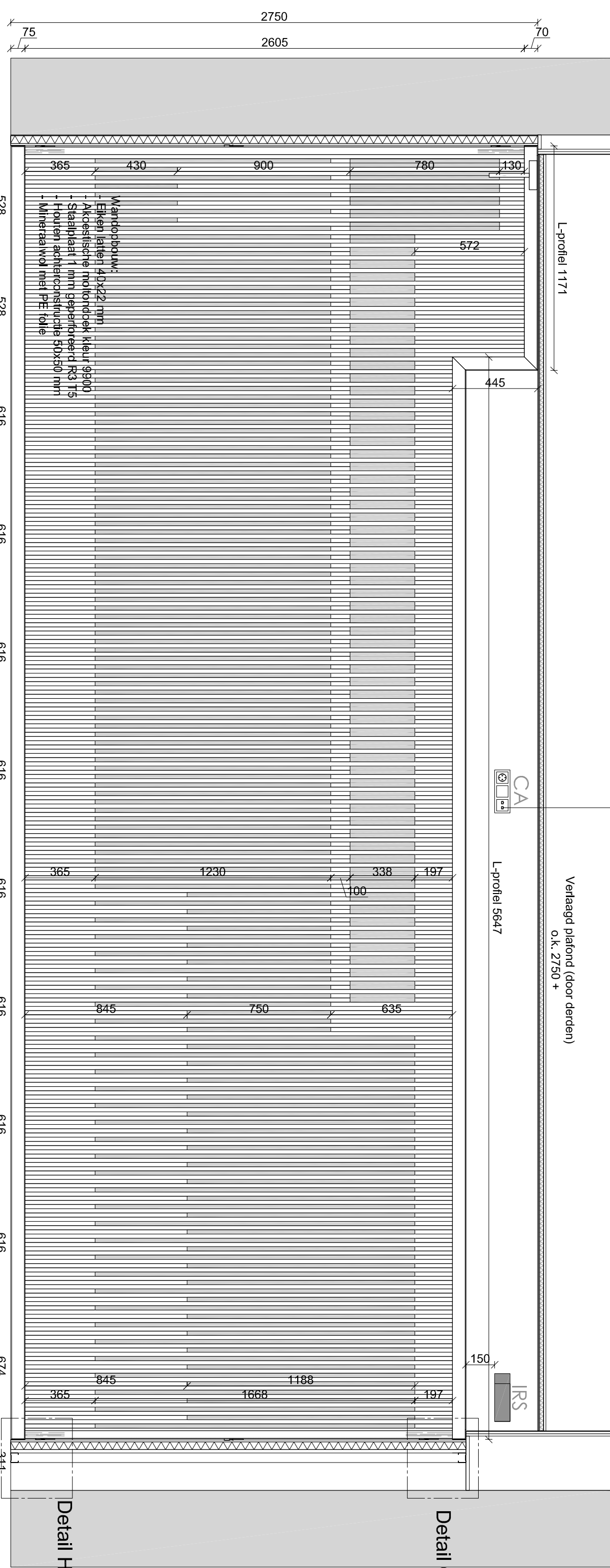
Aanzicht 1-1
