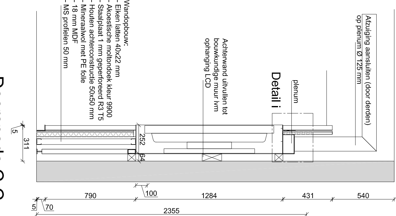
Doorsnede C-C
