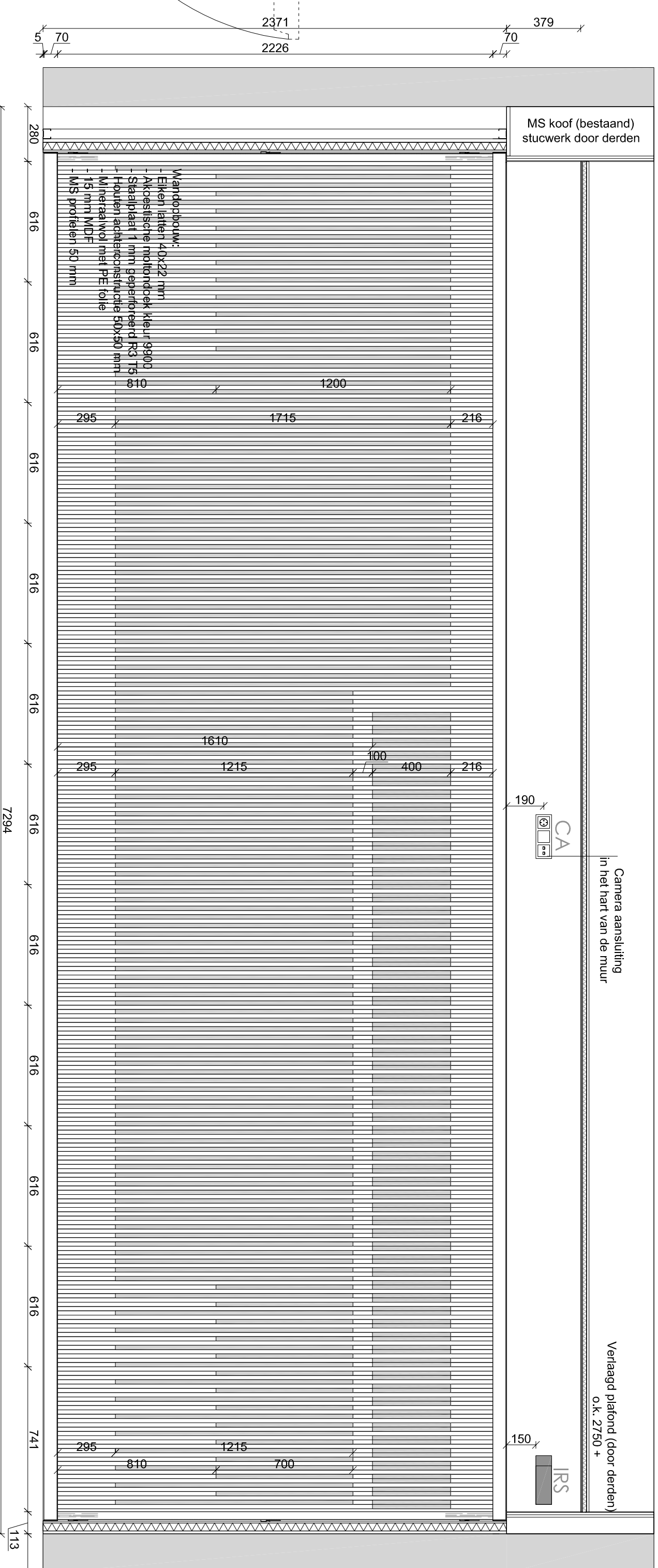
Aanzicht 2-2
