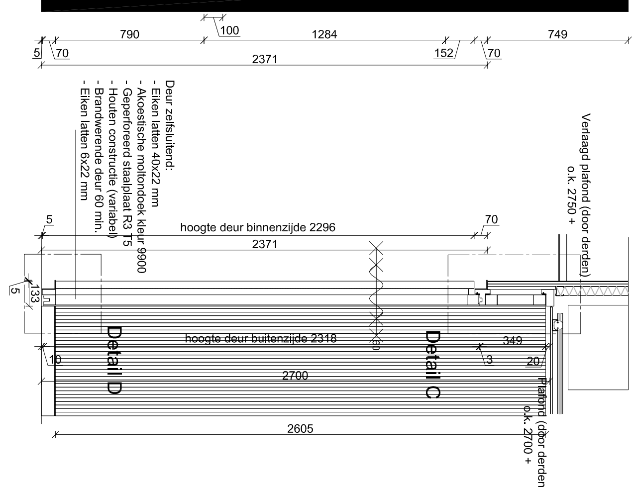
Doorsnede C-C
