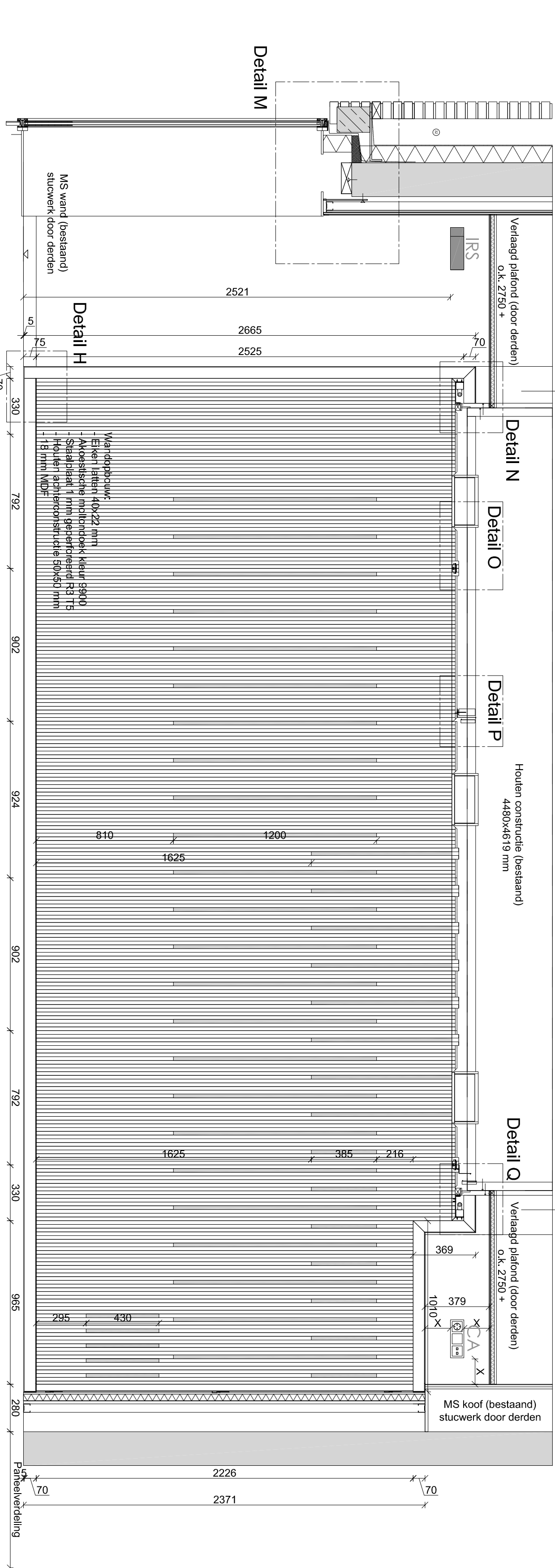
Aanzicht 1-1
