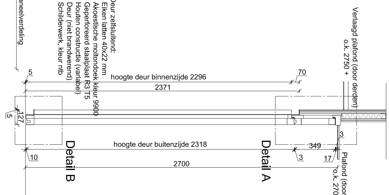
Doorsnede A-A
