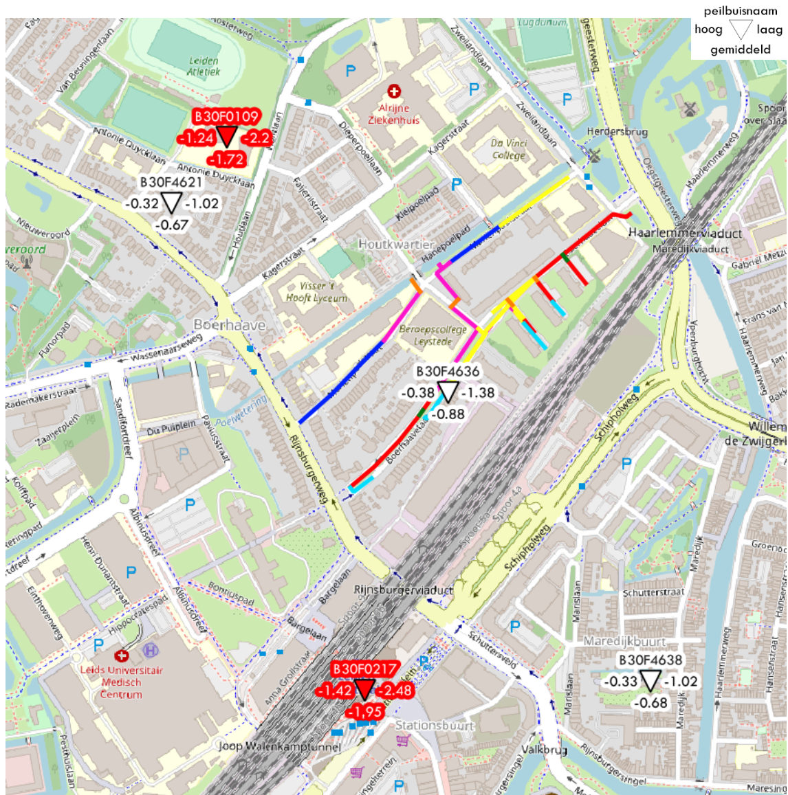
figuur 7 - grondwaterstand t.o.v. NAP per geanalyseerde peilbuis (wit = freatisch/watervoerende laag 1, rood = watervoerende laag 3)
