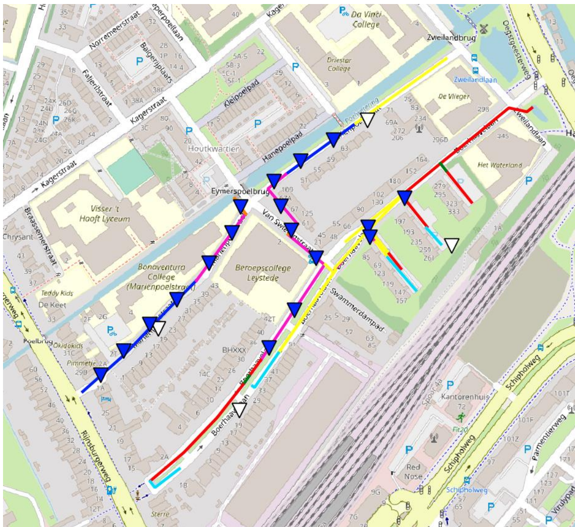
Figuur 6 - locatie peilbuizen (blauwe driehoek is voor instellen diepe filterbemaling, witte driehoeken zijn voor omgeving)
