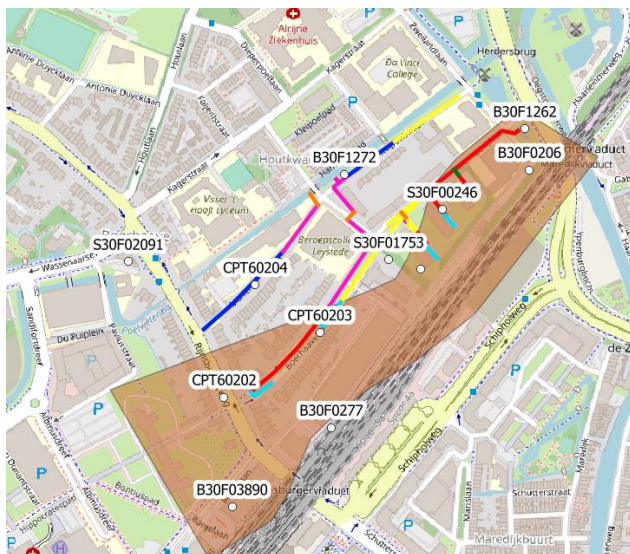
figuur 3 – locatie grondonderzoek (in het bruine vlak ontbreekt watervoerende laag 2)
