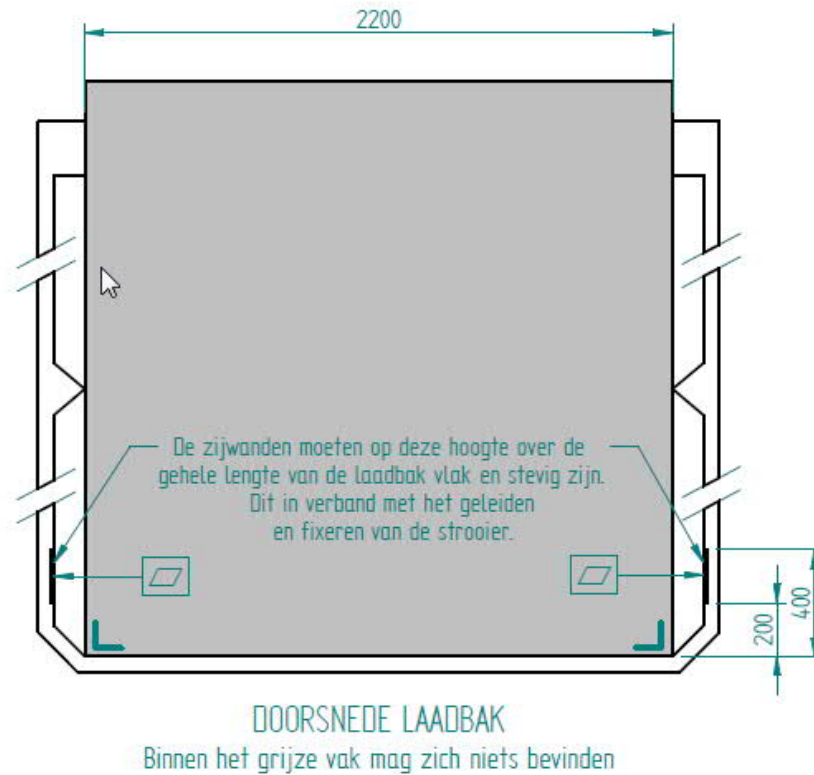
Figuur 2: doorsnede laadbak
