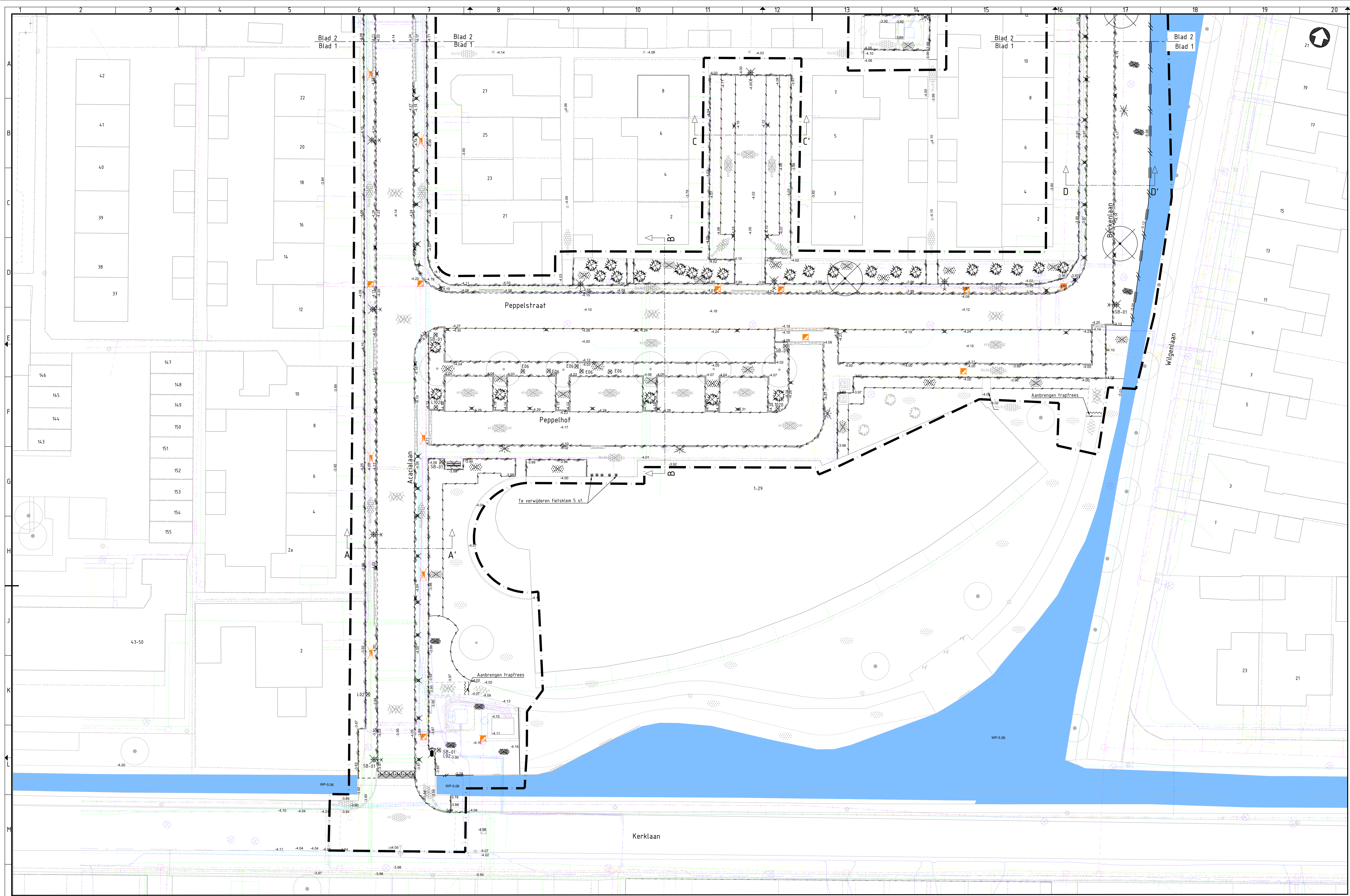
KADER 1 BESTAANDE SITUATIE K&L SCHAAL 1 : 200
