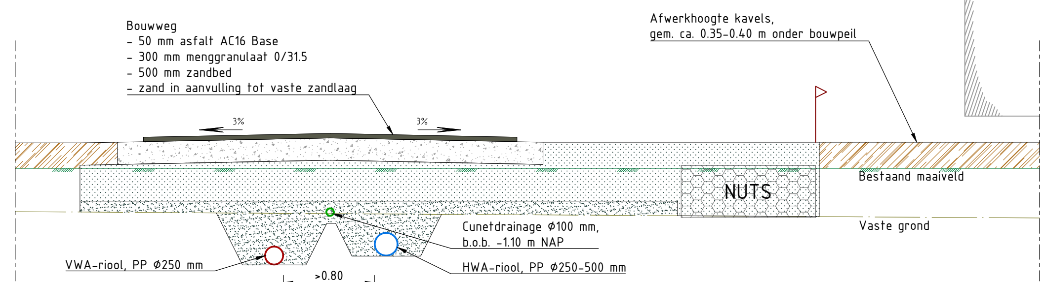
Principeprofiel BRM
