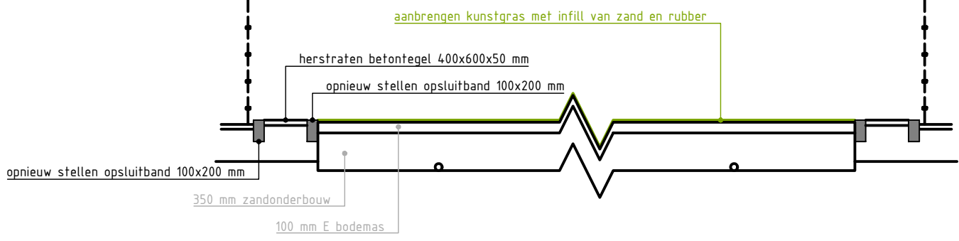
principeddoorsnede veld SCHAAL 1 : 50
