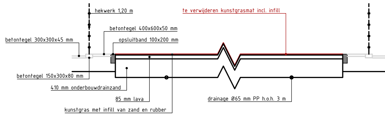
principeddoorsnede veld SCHAAL 1 : 50
