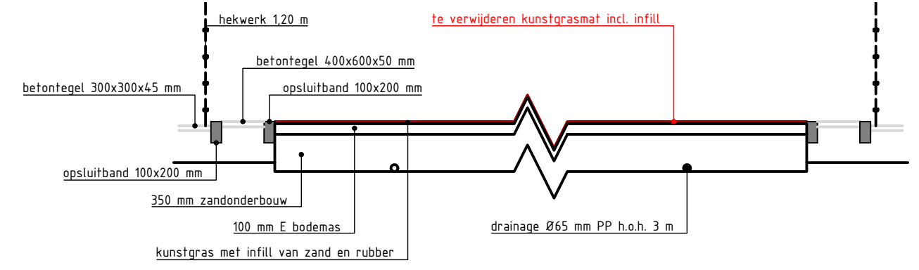
principeddoorsnede veld SCHAAL 1 : 50
