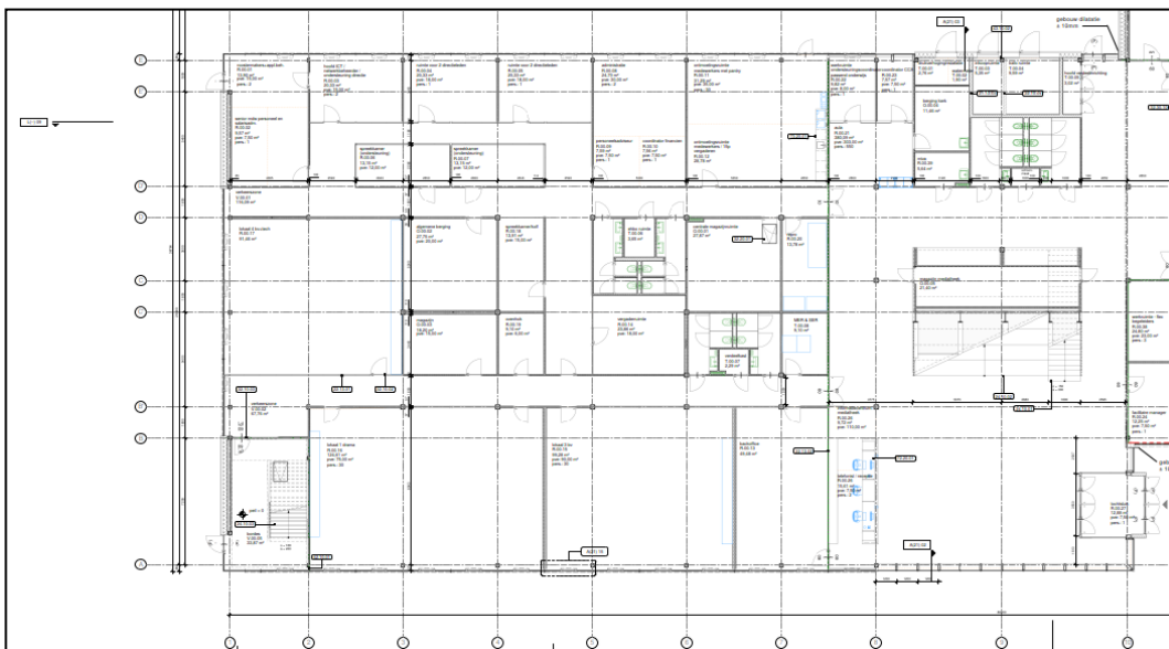
Figuur 4 Fragment van de linker gebouwleugel (plattegrond begane grond uit het Definitief Ontwerp). Nog geen bestek.
