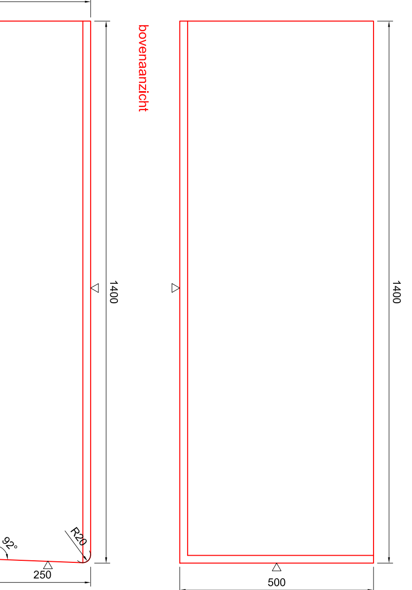
Merk TR04 R trapreus, rechts 1400/1390x500/490x250mm
