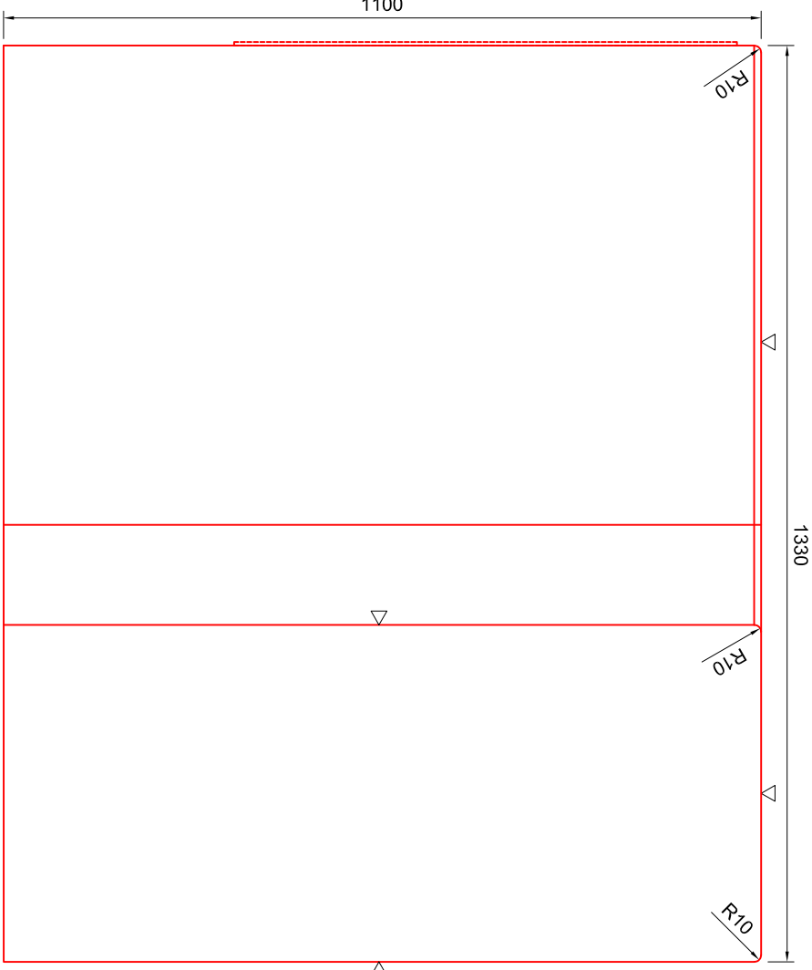
Merk KIM5 keermuur, hoekstuk 102° 1000x500x1000mm
