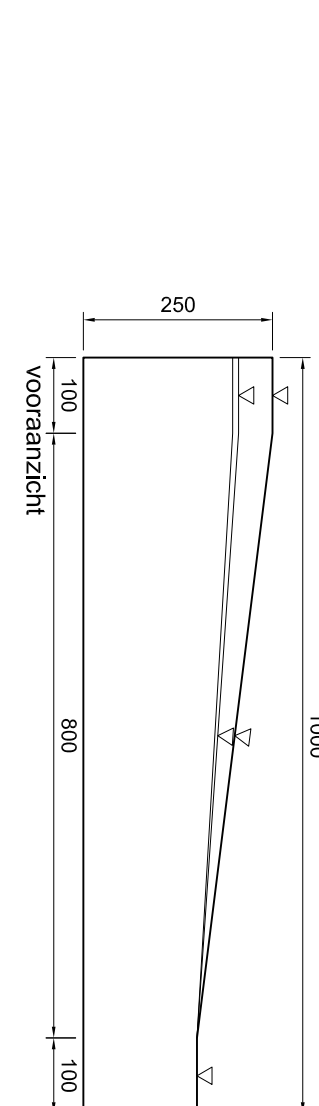
Merkb01 R Eindevelopband GB5/20, rechts 1000x300x250/100mm
