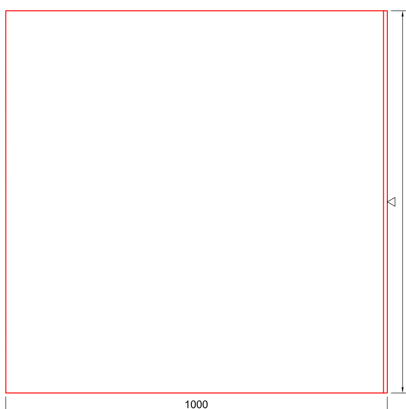
Merk KIM6 muur 1000x405x1000mm
