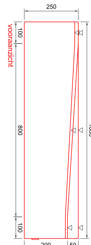
Merkb04 R Verlooptband TB30 naar GB5/20, rechts 1000x300/200x250mm
