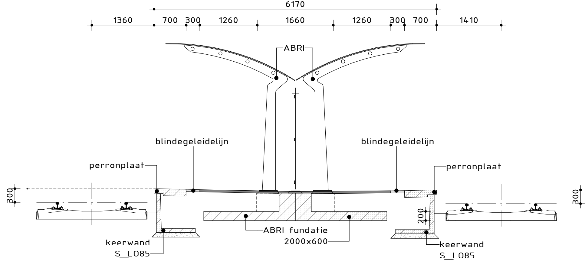
Dwarsdoorsnede A Schaal 1 : 50
