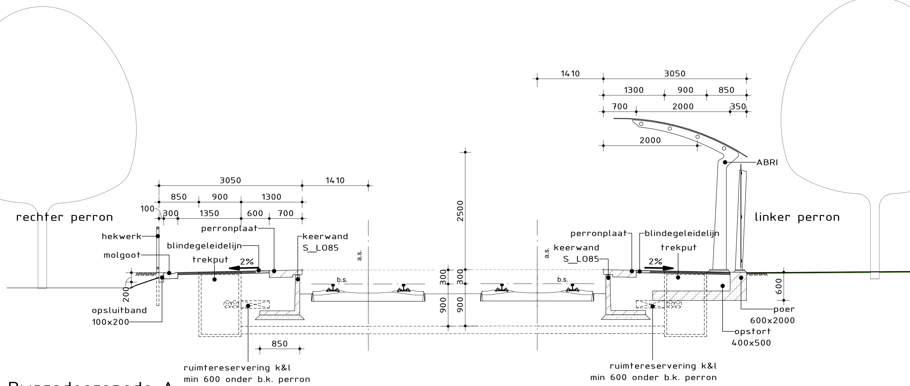
Dwarsdoorsnede A
