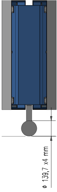
Bovenaanzicht
