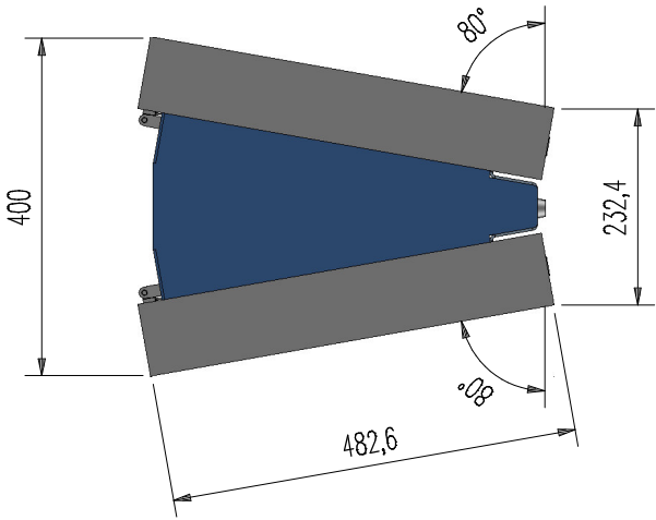
Zijraanzicht
