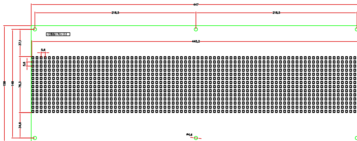
Vooraanzicht
