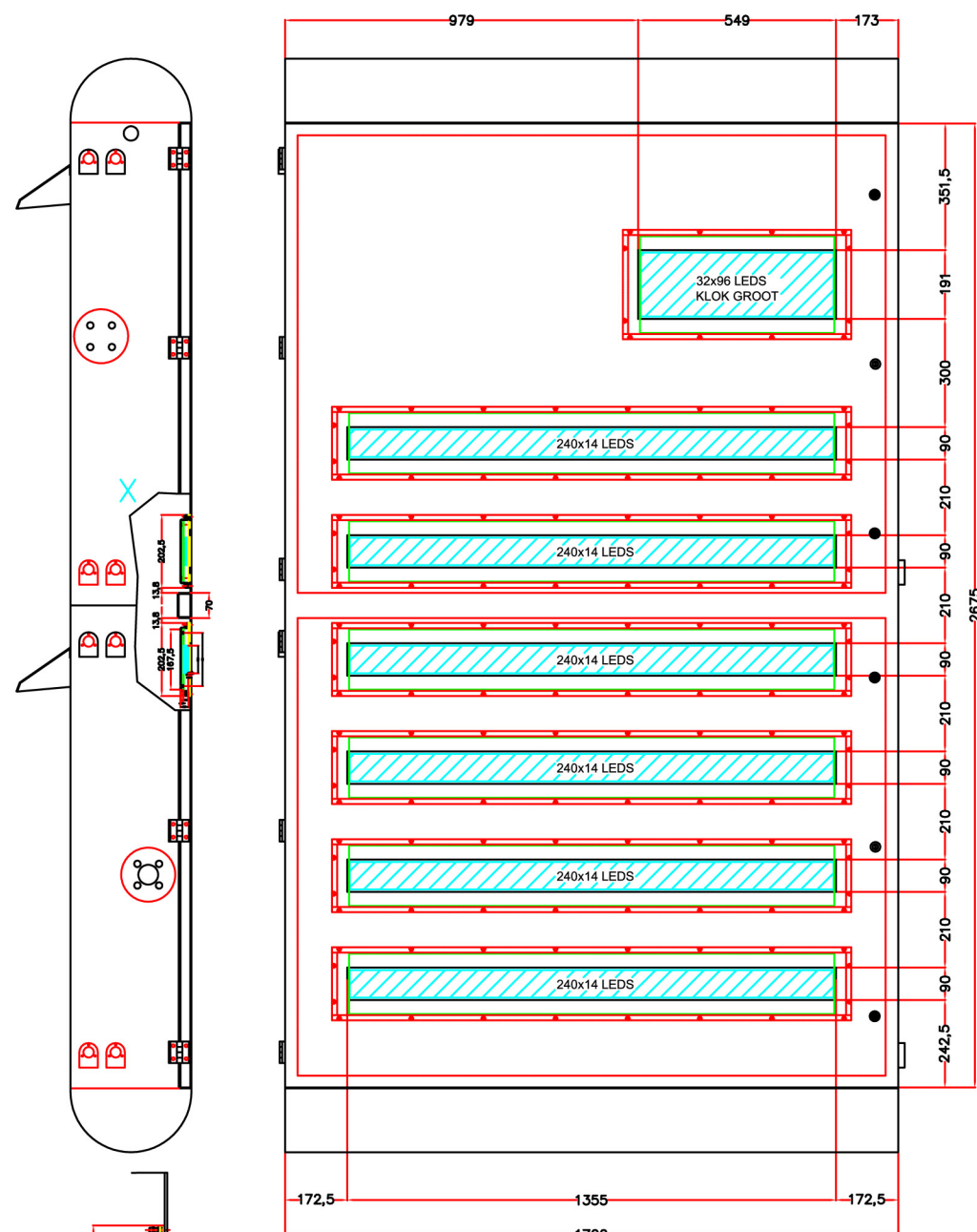
Vooraanzicht
