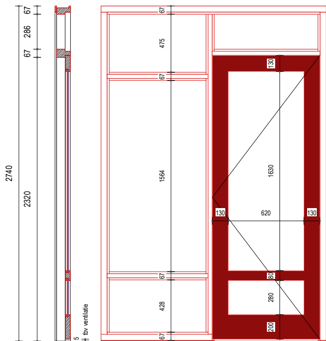
KOZIJNMERK Bi.K.01.12 : - aantal : 1 st.
