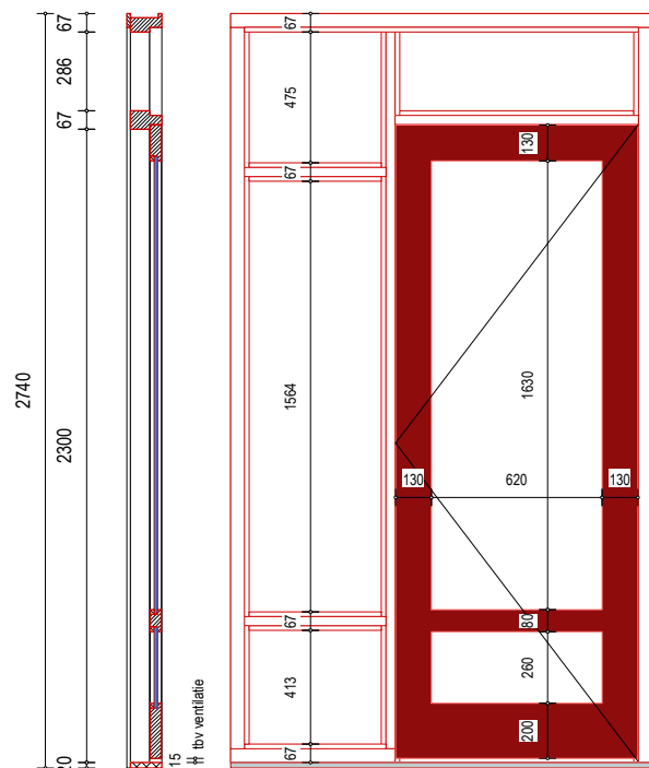
KOZIJNMERK Bi.K.01.13.1/2: - aantal : 2 st.
