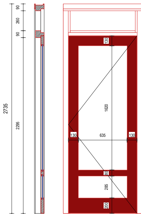
KOZIJNMERK Bi.K.01.17 ( 30 min. WBDBO ): - aantal : 1 st.
