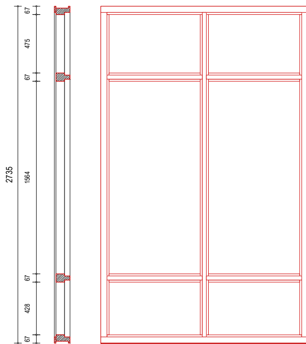
KOZIJNMERK Bi.K.01.16 : - aantal : 1 st.
