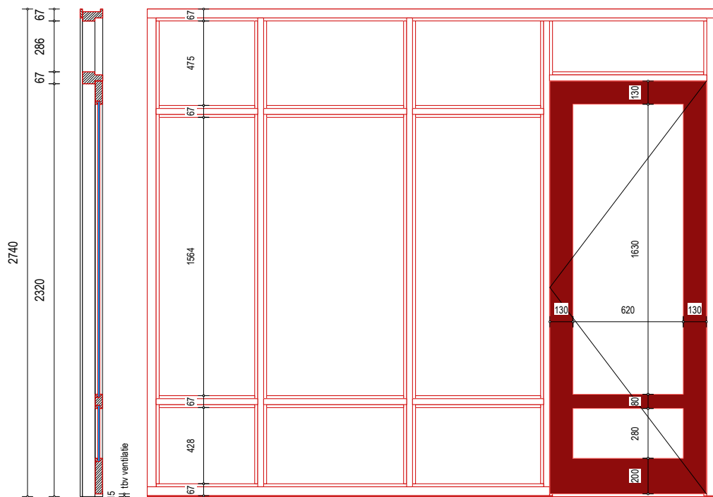
KOZIJNMERK Bi.K.01.15 : - aantal : 1 st.
