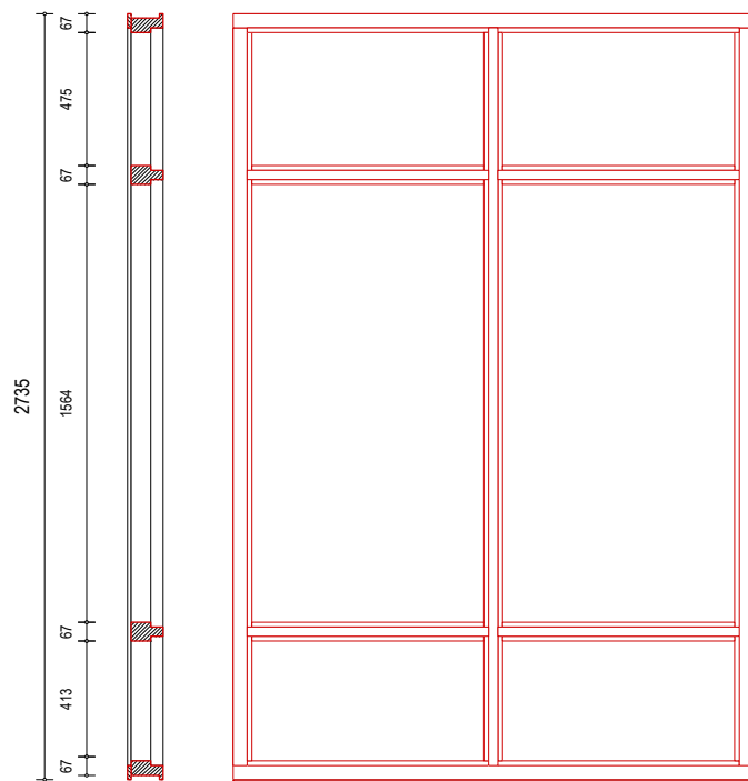
KOZIJNMERK Bi.K.01.14 : - aantal : 1 st.
