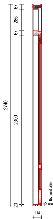
KOZIJNMERK Bi.K.01.05.1/2: - aantal : 2 st.
