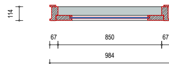
KOZIJNMERK Bi.K.01.04.1/2/3 : - aantal : 2 st. als getekend 1 st. gespiegeld - deur : 40mm, stomp - vulling : glas - kozijnen : hout
