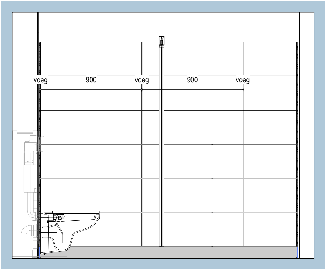
DOORSNEDE B-B
