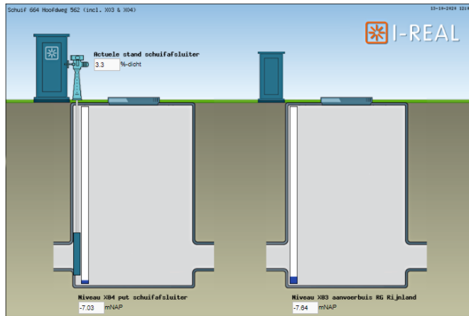
Schuif 664 Hoofdweg 562 (incl. X03 & X04): Schematische weergave
