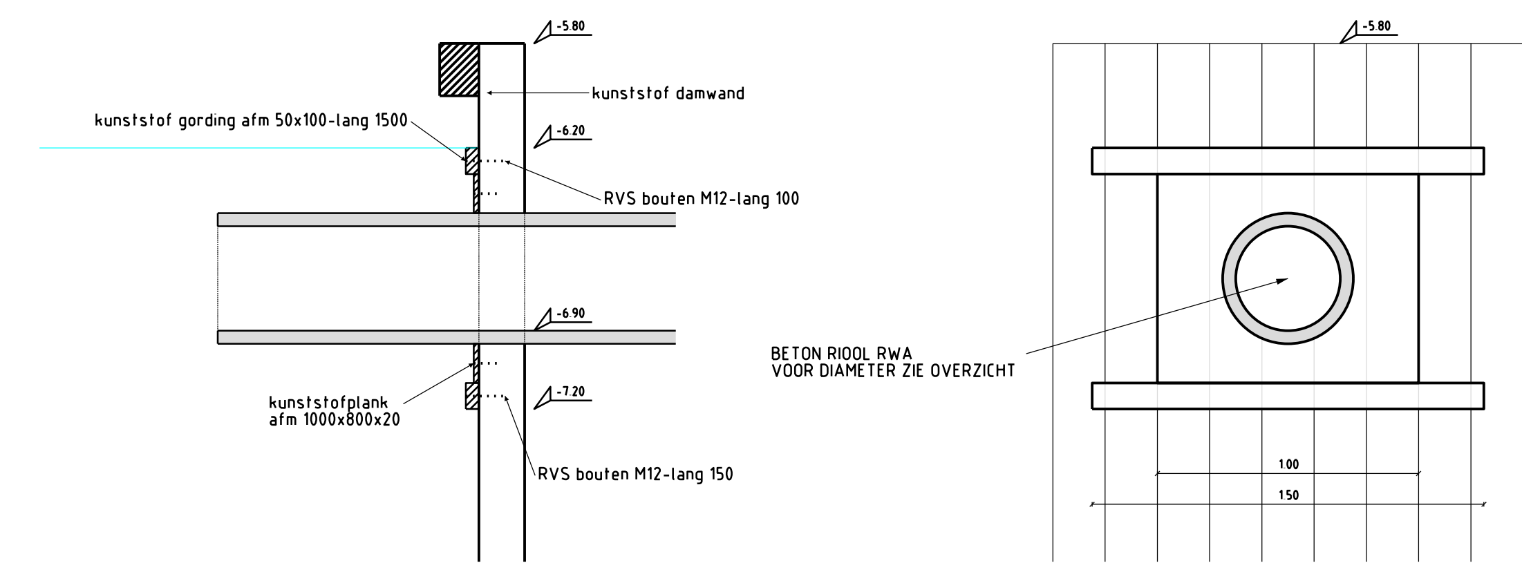
Aanbrengen uitmonding RWA riool Schaal 120
