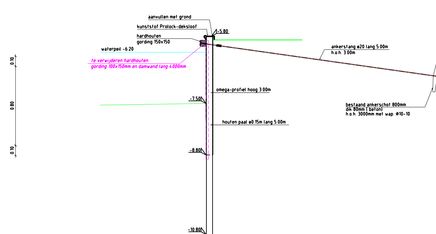
Principe profiel 1 vervang beschoeiing Schaal 150
