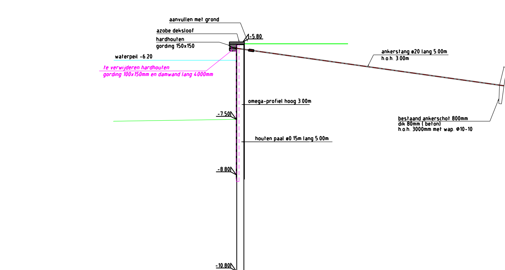
Principe profiel 2 vervang beschoeiing Schaal 150
