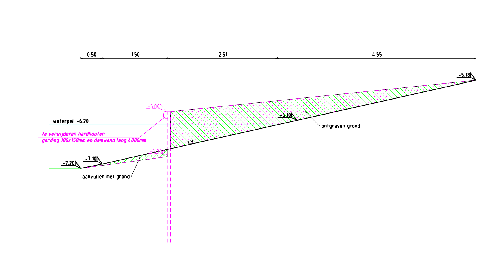
Principe profiel 3 natuurvriendelijke oevers Schaal 150
