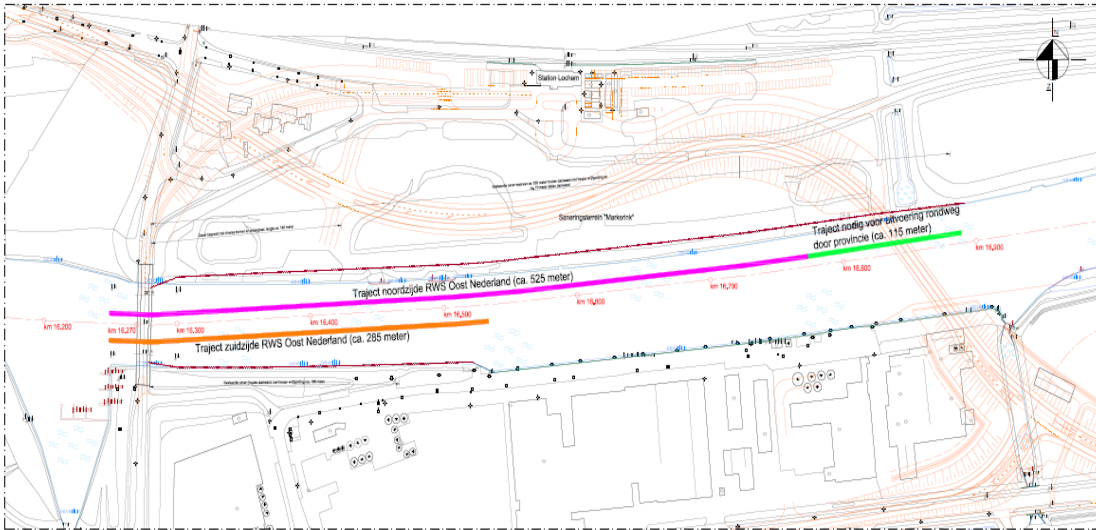
Situatie Verruiming vaargeul t.p.v. Markerink te Lochem
