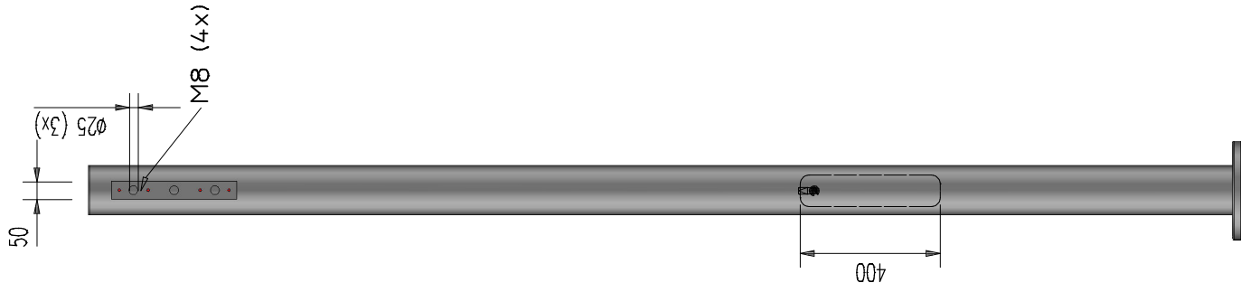
Zijraanzicht
