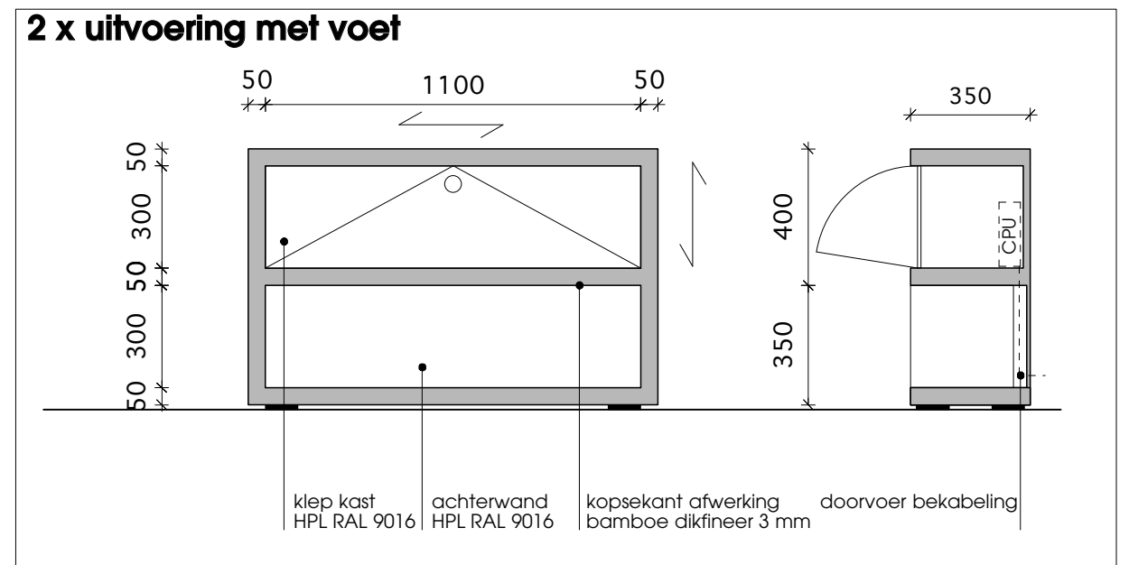
doorsnede A - A'
