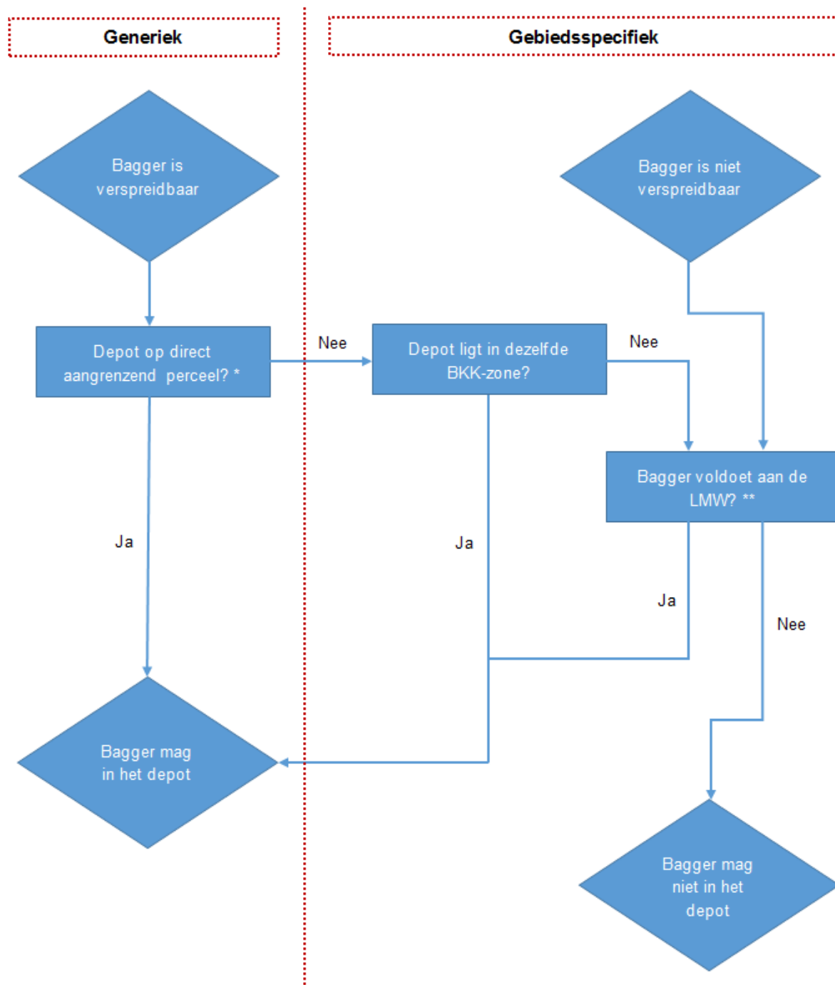
Figuur 6.4: beslisschema weilanddepots.
